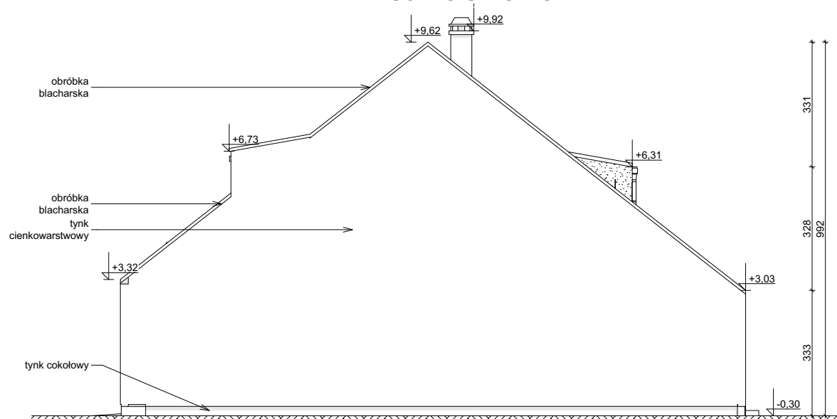
ELEWACJA BOCZNA
