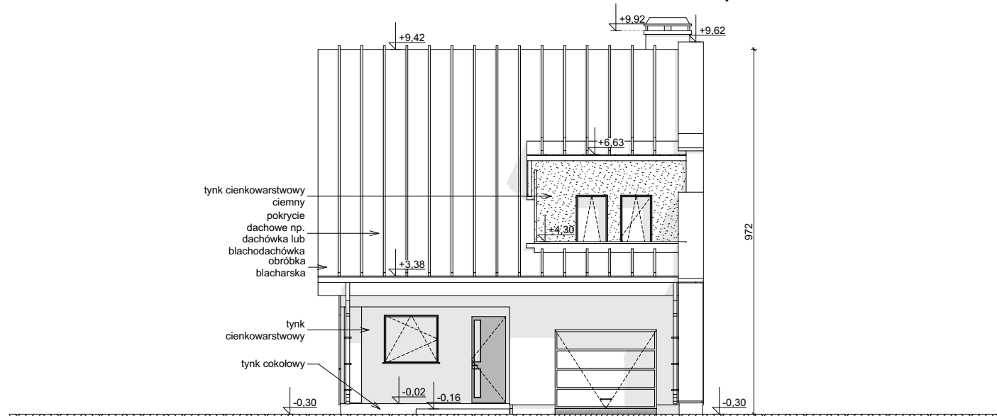
ELEWACJA FRONTOWA
