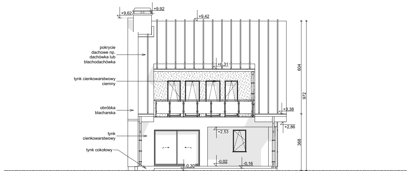
ELEWACJA OGRODOWA
