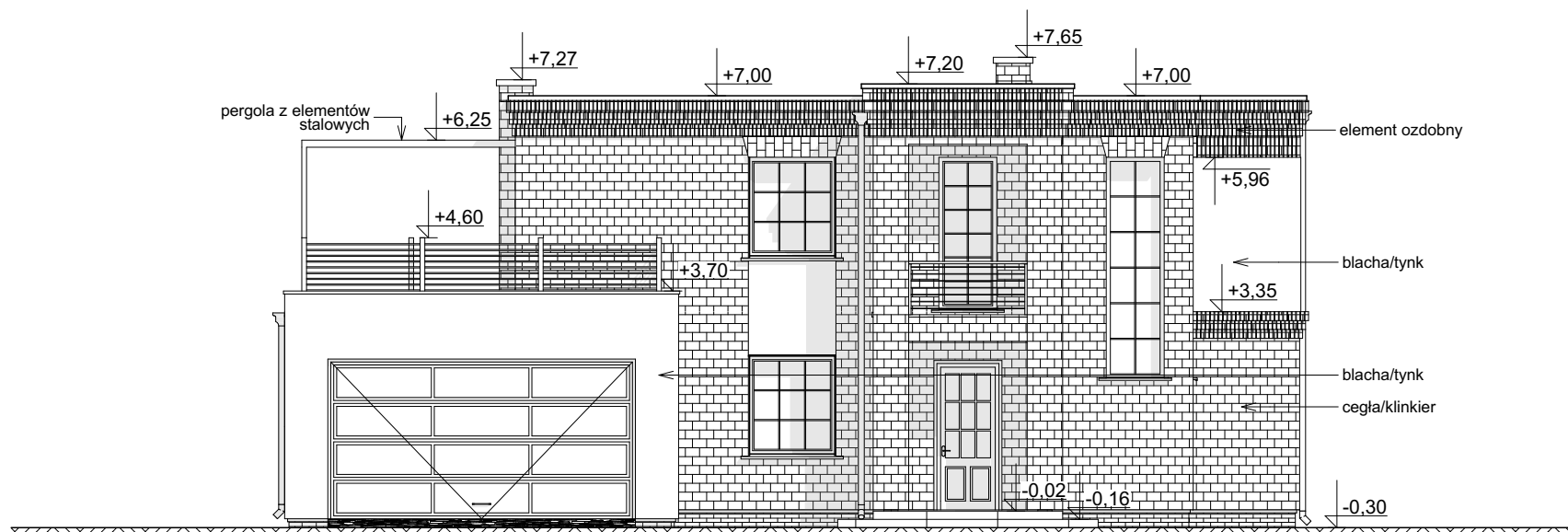
ELEWACJA FRONTOWA
