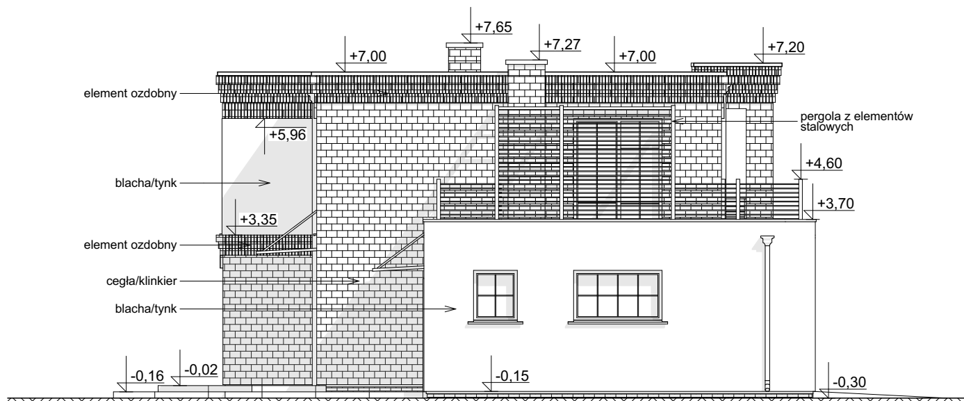
ELEWACJA BOCZNA
