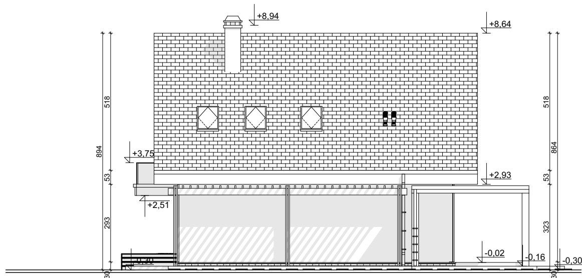
ELEWACJA BOCZNA
