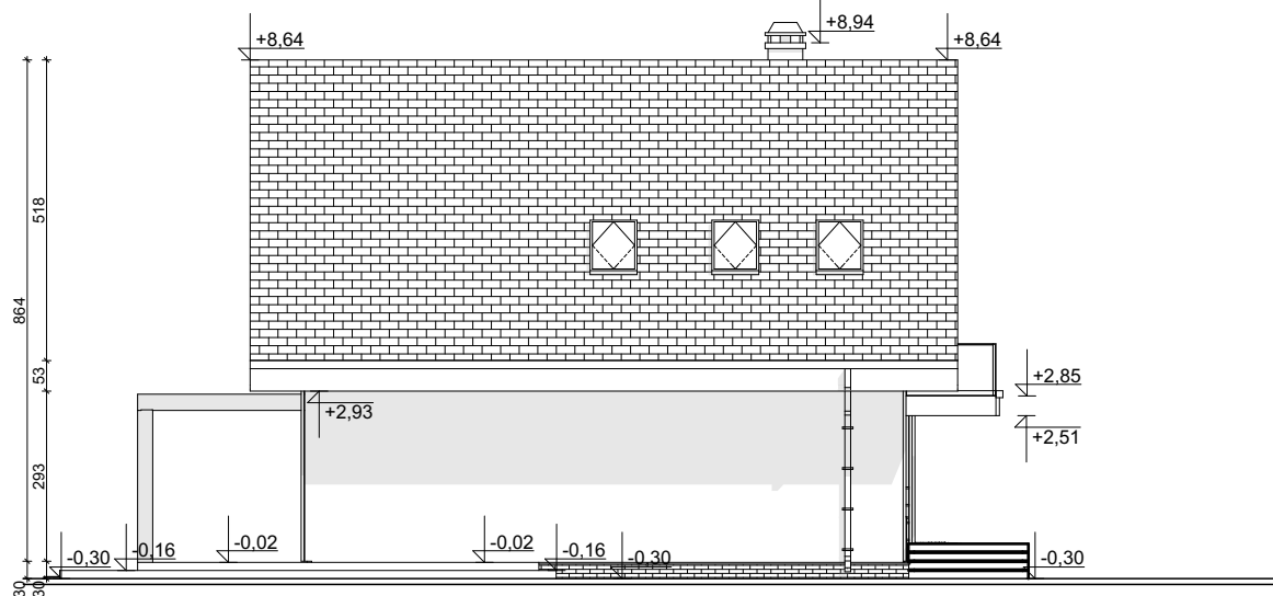
ELEWACJA BOCZNA
