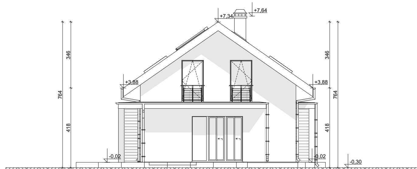
ELEWACJA BOCZNA
