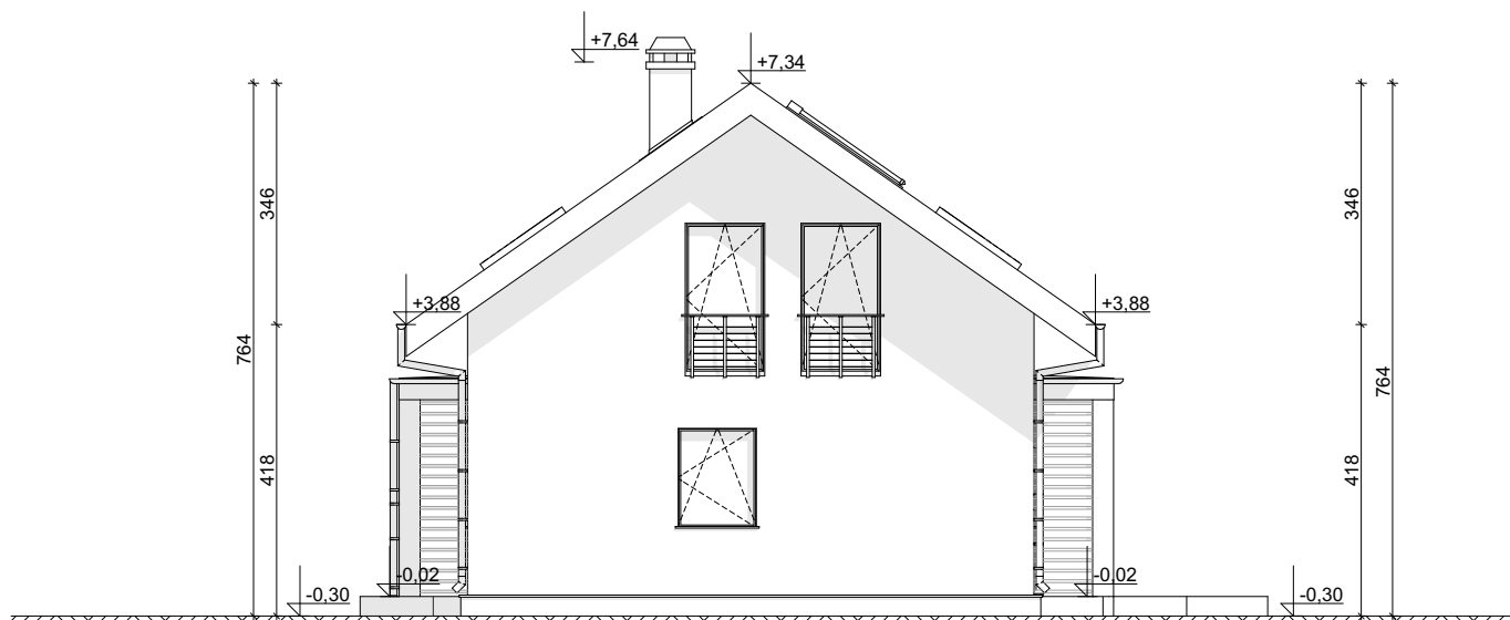
ELEWACJA BOCZNA
