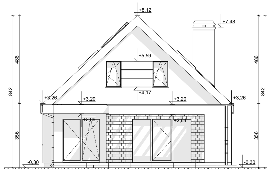
ELEWACJA OGRODOWA
