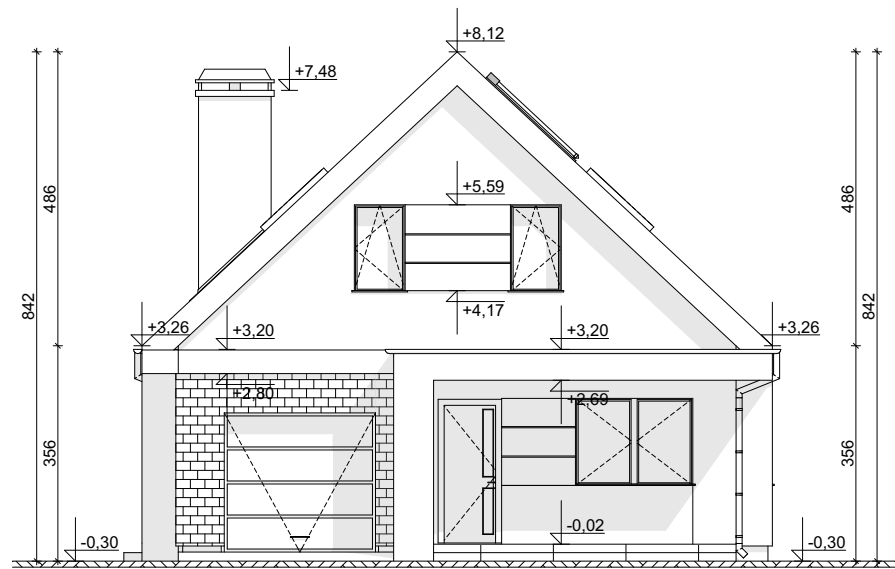
ELEWACJA FRONTOWA
