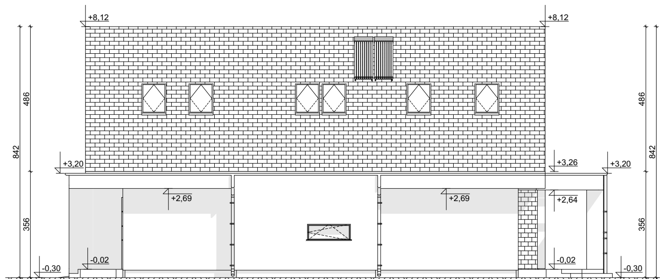
ELEWACJA BOCZNA
