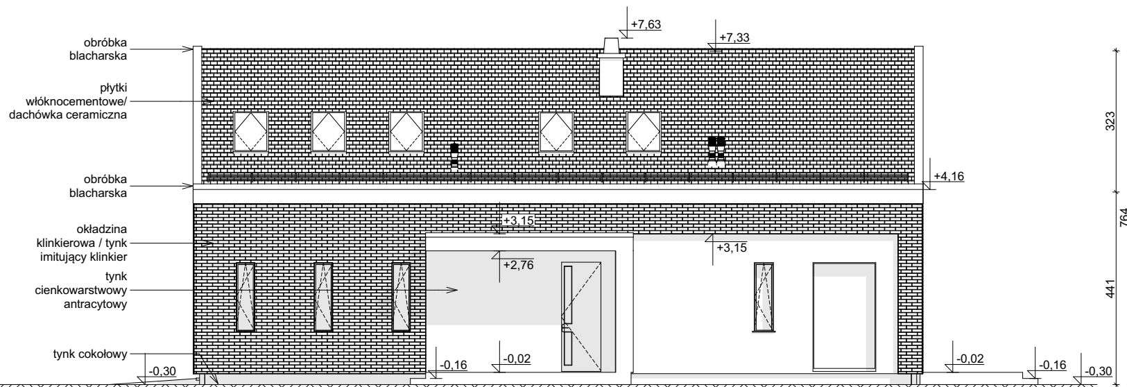
ELEWACJA FRONTOWA
