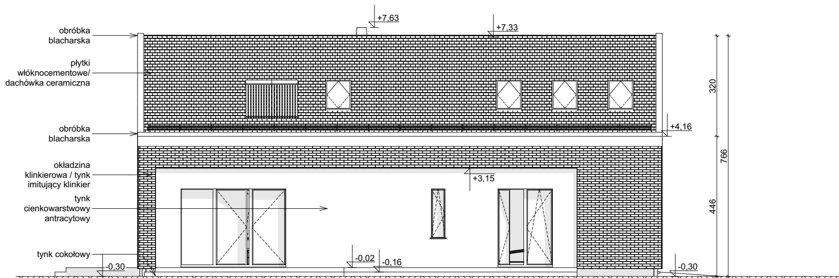
ELEWACJA OGRODOWA
