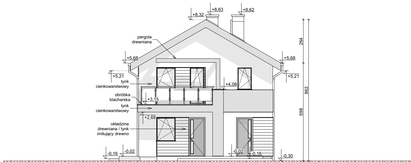
ELEWACJA FRONTOWA
