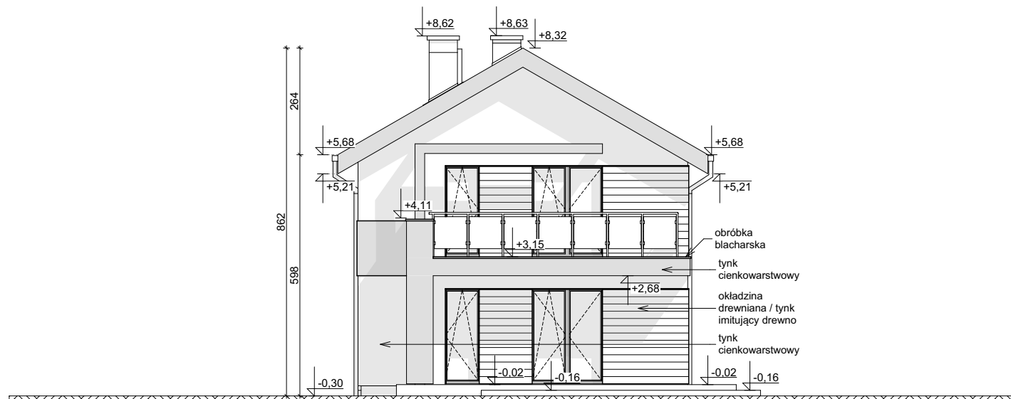
ELEWACJA OGRODOWA
