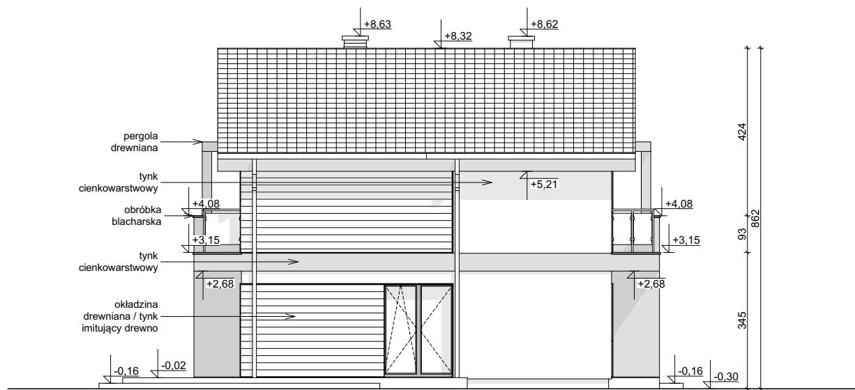
ELEWACJA BOCZNA
