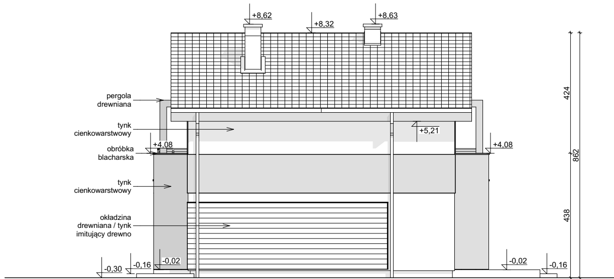
ELEWACJA BOCZNA
