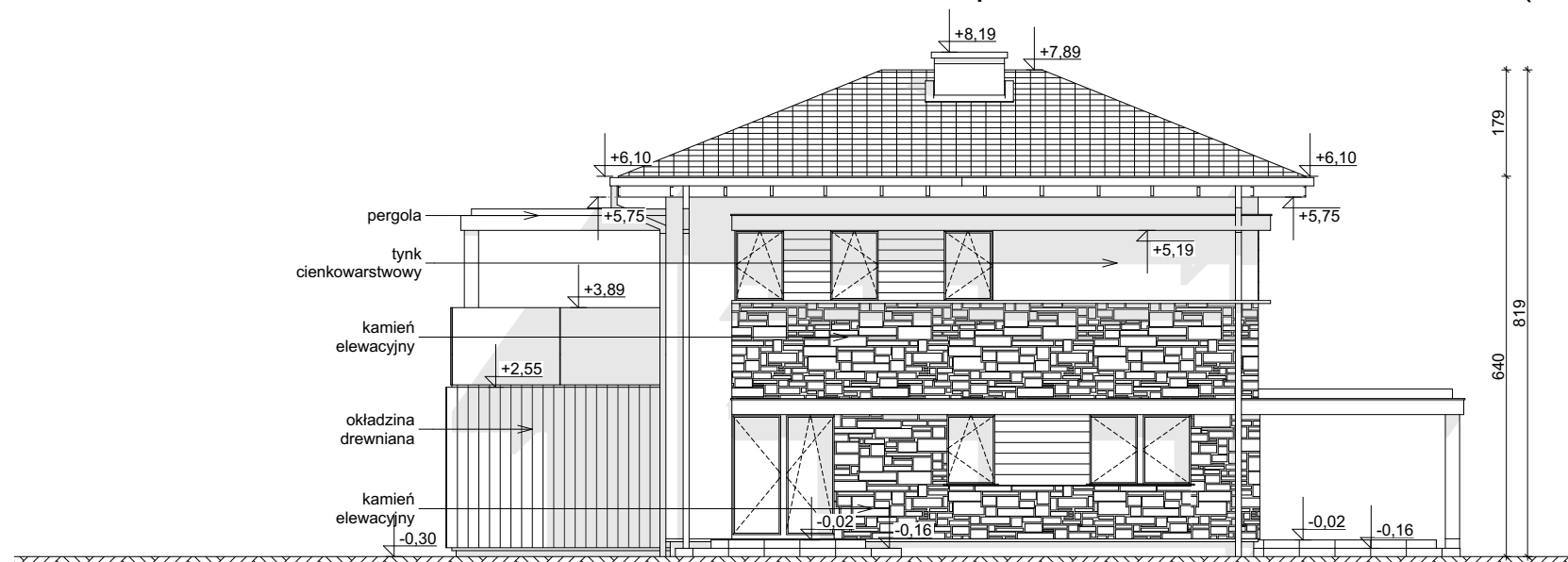
ELEWACJA OGRODOWA
