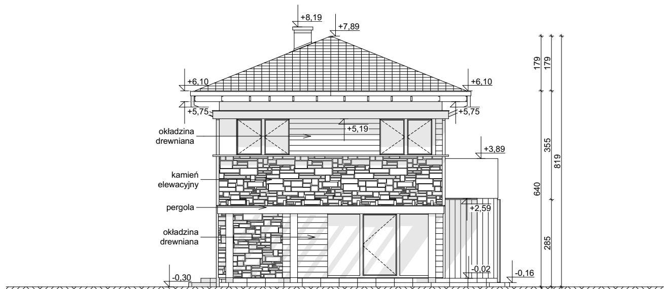
ELEWACJA BOCZNA
