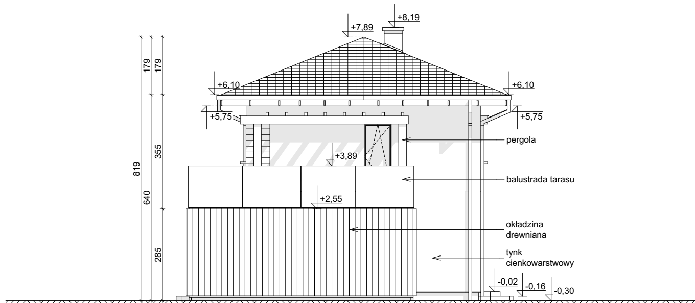
ELEWACJA BOCZNA
