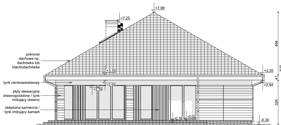
ELEWACJA OGRODOWA
