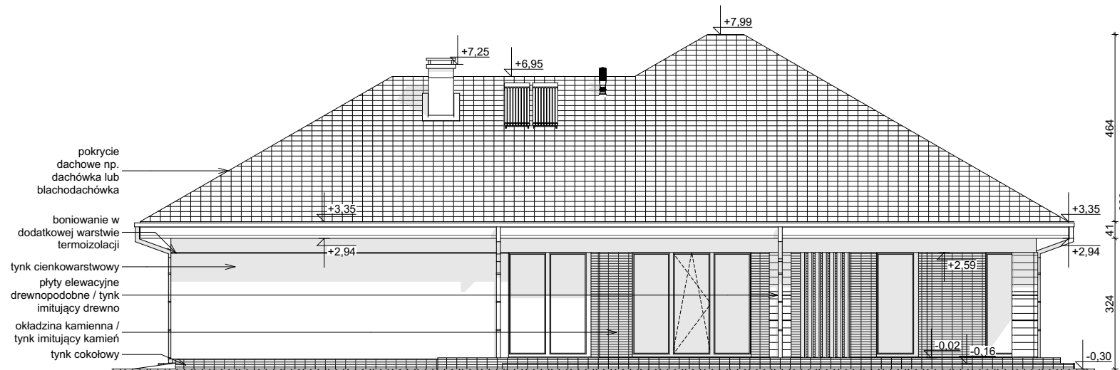
ELEWACJA BOCZNA
