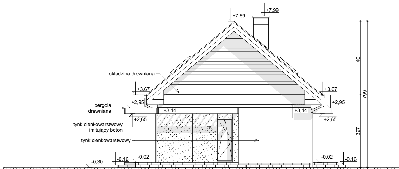
ELEWACJA BOCZNA
