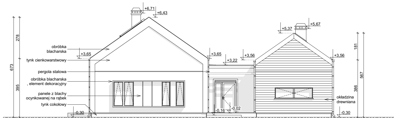
ELEWACJA FRONTOWA
