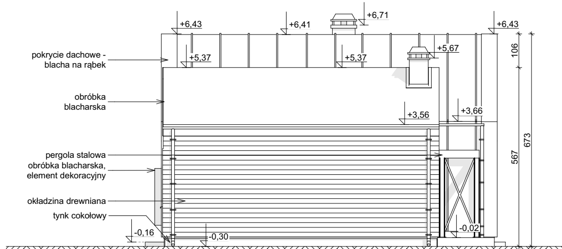
ELEWACJA BOCZNA
