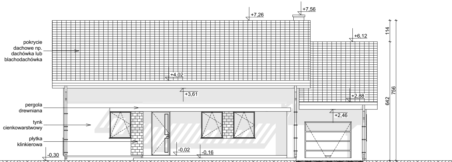
ELEWACJA FRONTOWA
