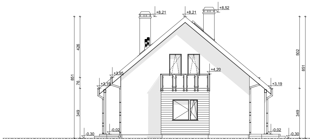
ELEWACJA BOCZNA
