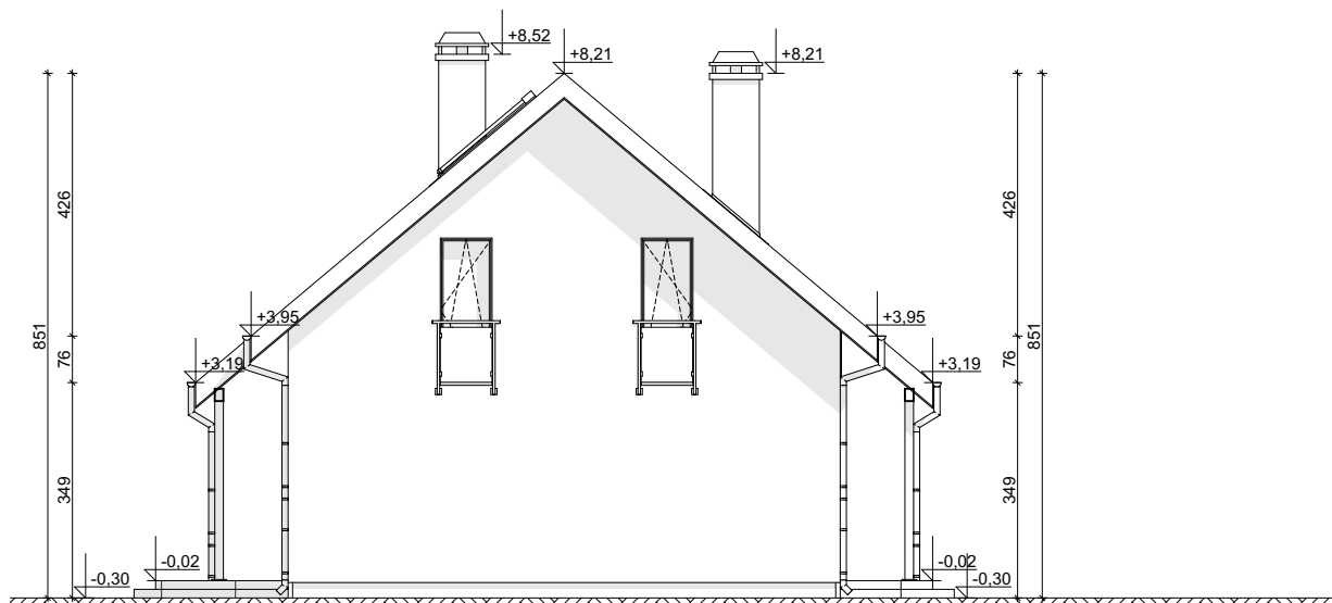
ELEWACJA BOCZNA
