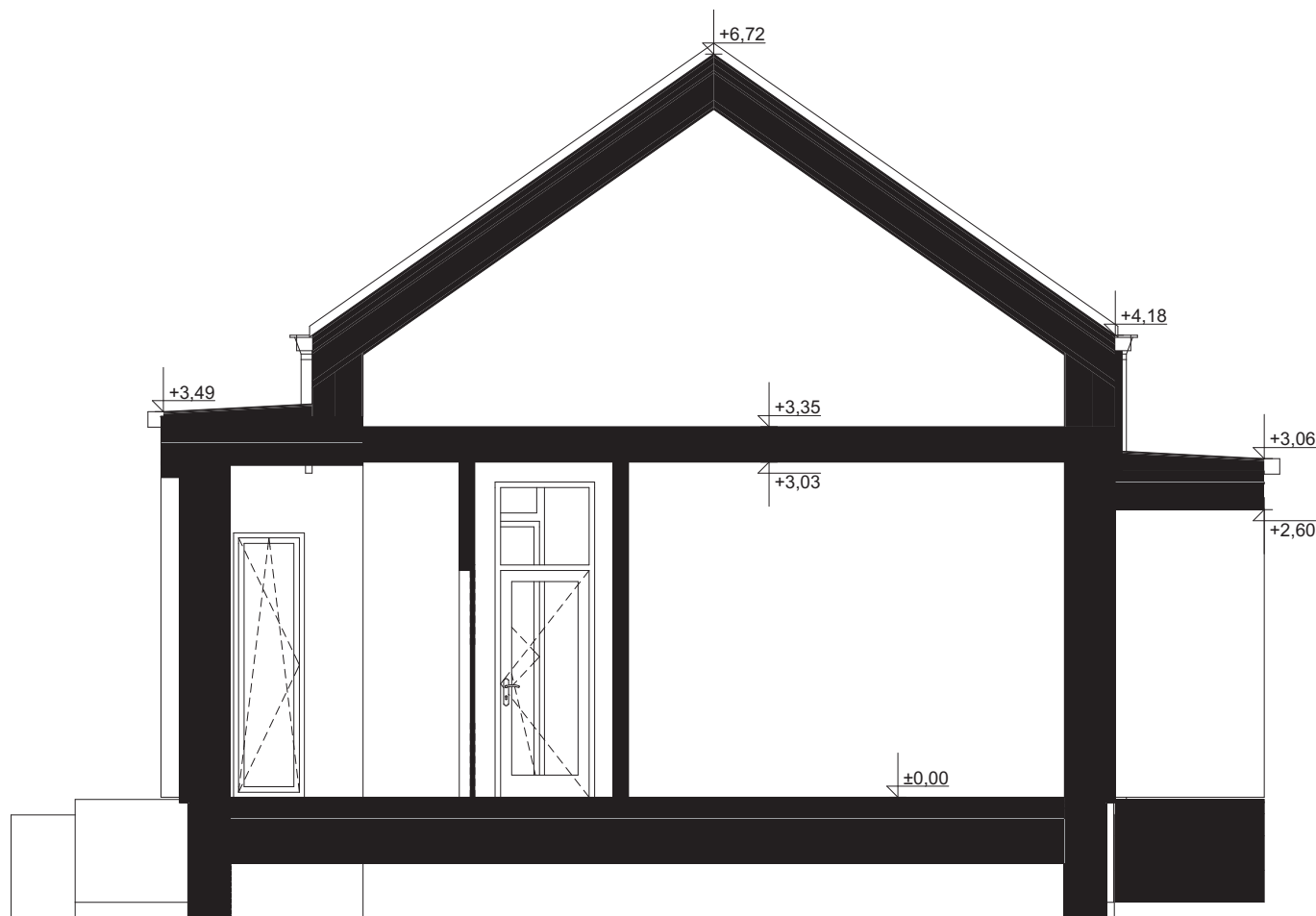
A-A
