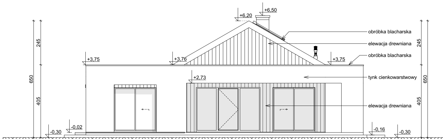
ELEWACJA OGRODOWA
