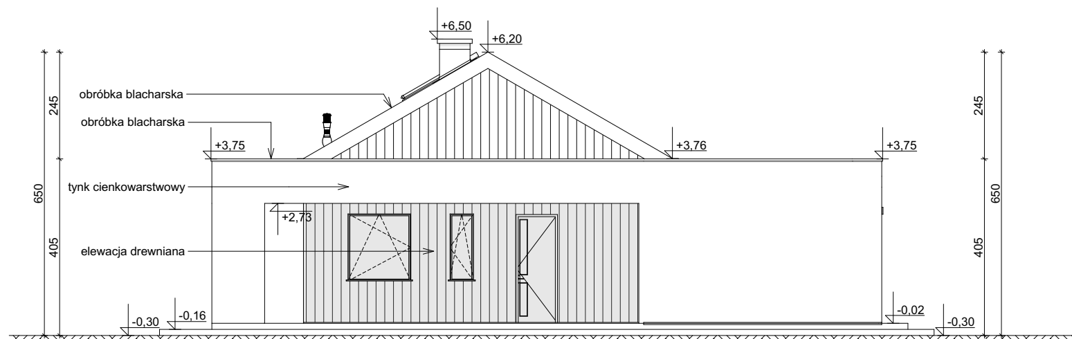
ELEWACJA FRONTOWA
