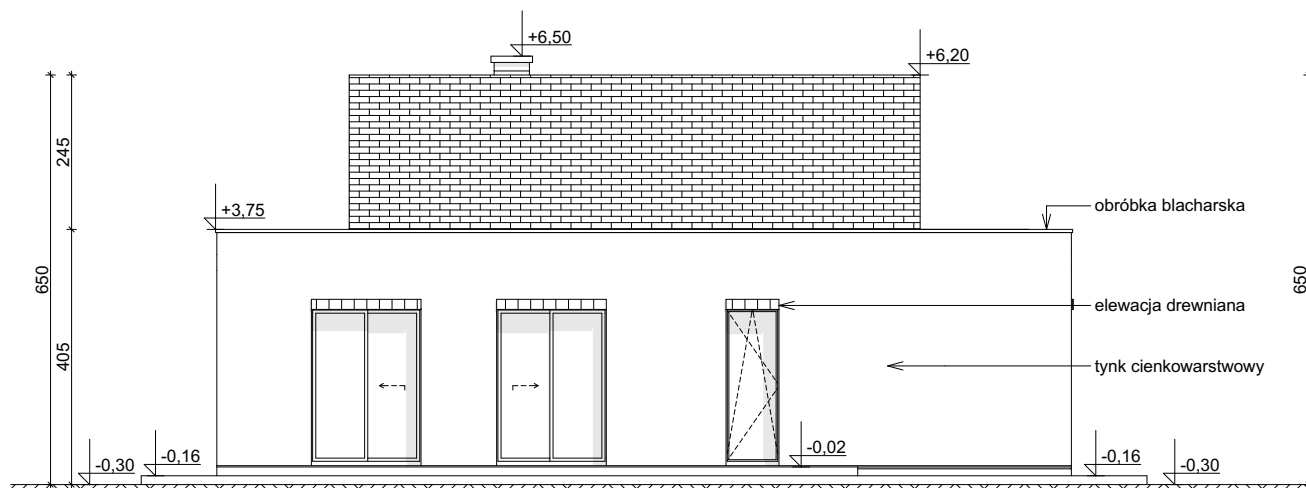
ELEWACJA BOCZNA
