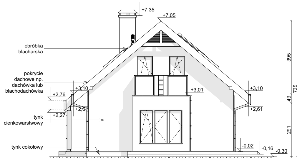
ELEWACJA BOCZNA
