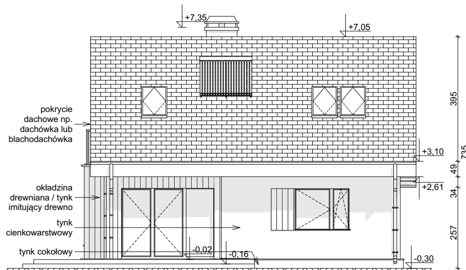
ELEWACJA OGRODOWA
