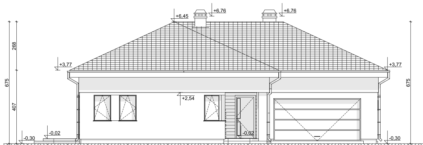
ELEWACJA FRONTOWA
