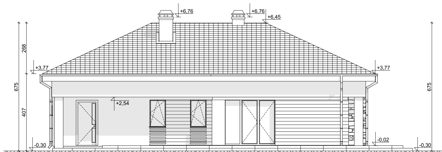
ELEWACJA OGRODOWA
