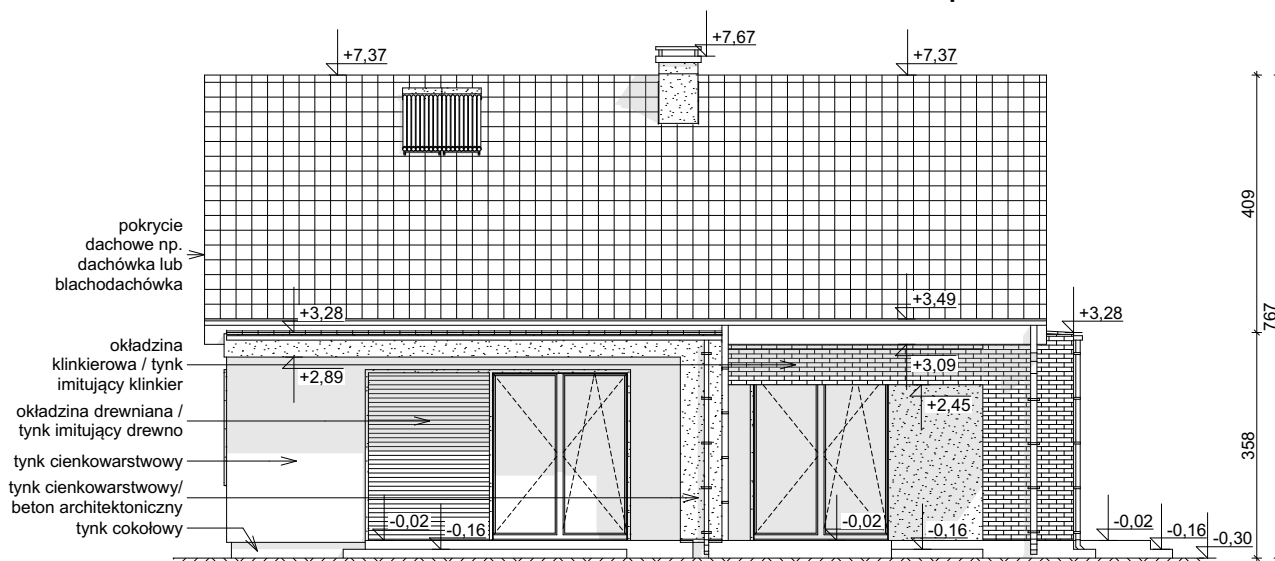
ELEWACJA OGRODOWA
