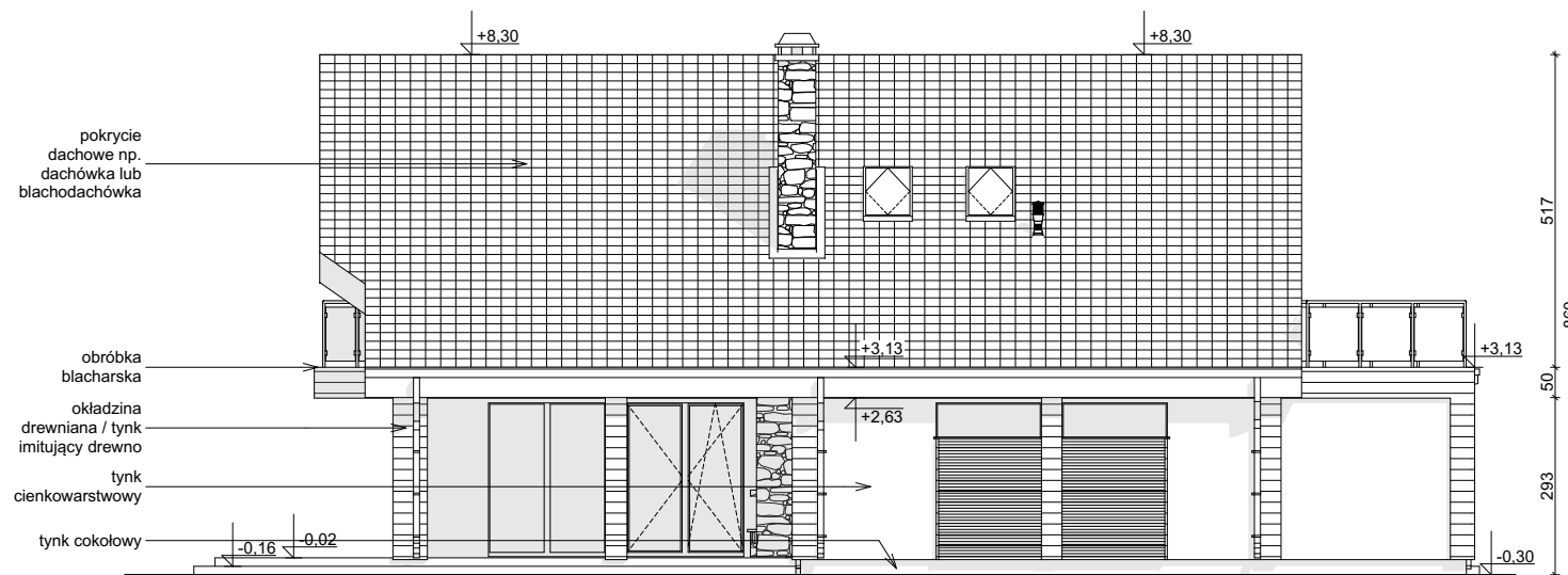
ELEWACJA BOCZNA
