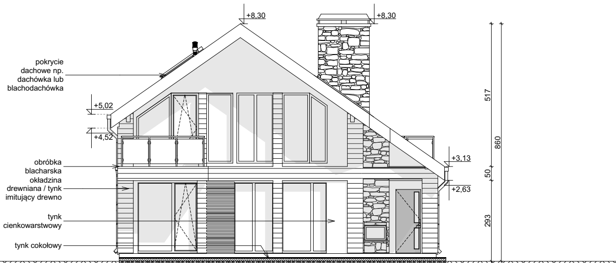
ELEVACJA OGRODOWA
