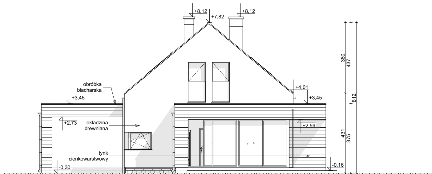
ELEWACJA OGRODOWA
