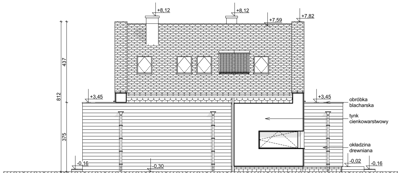
ELEWACJA BOCZNA
