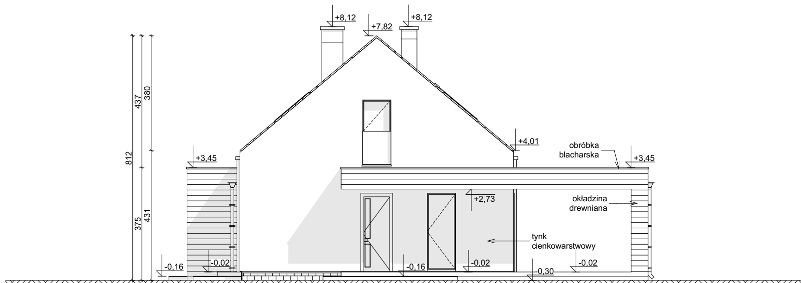
ELEWACJA FRONTOWA
