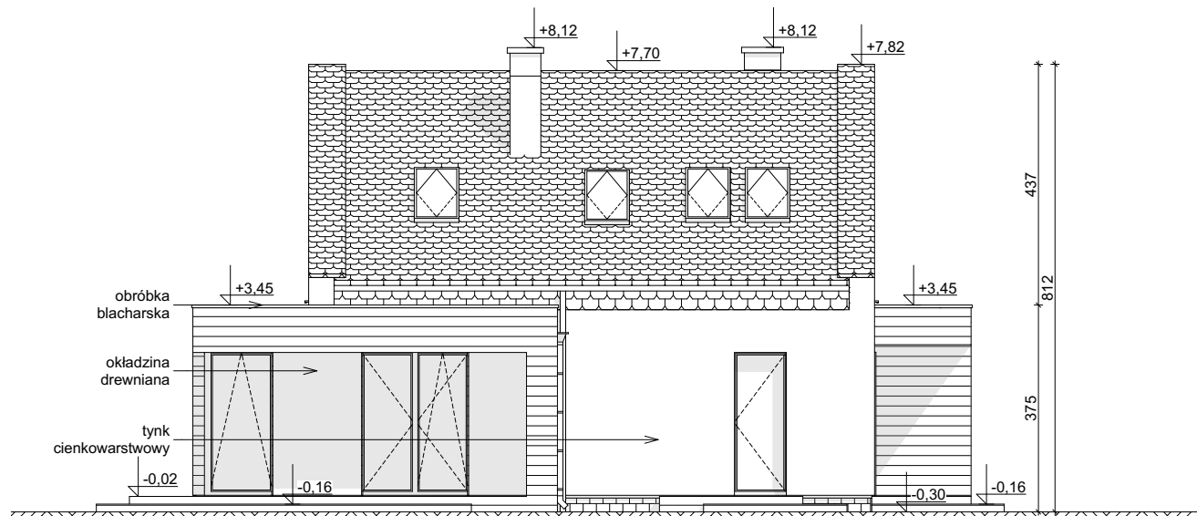
ELEWACJA BOCZNA
