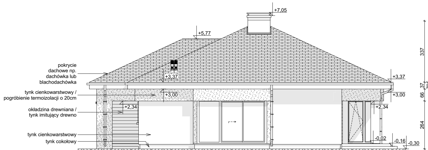
ELEWACJA BOCZNA
