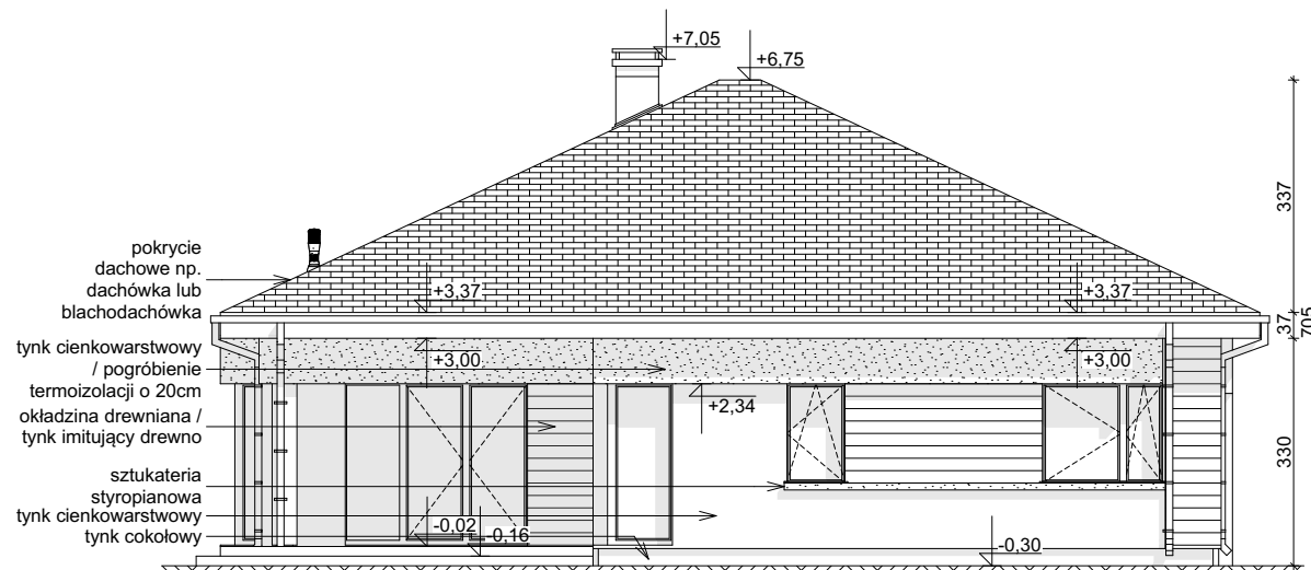
ELEWACJA OGRODOWA
