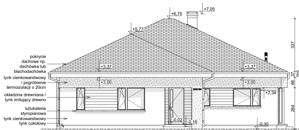
ELEWACJA FRONTOWA
