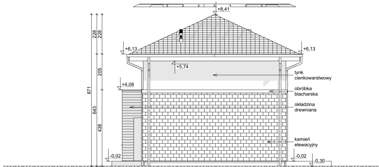
ELEWACJA BOCZNA
