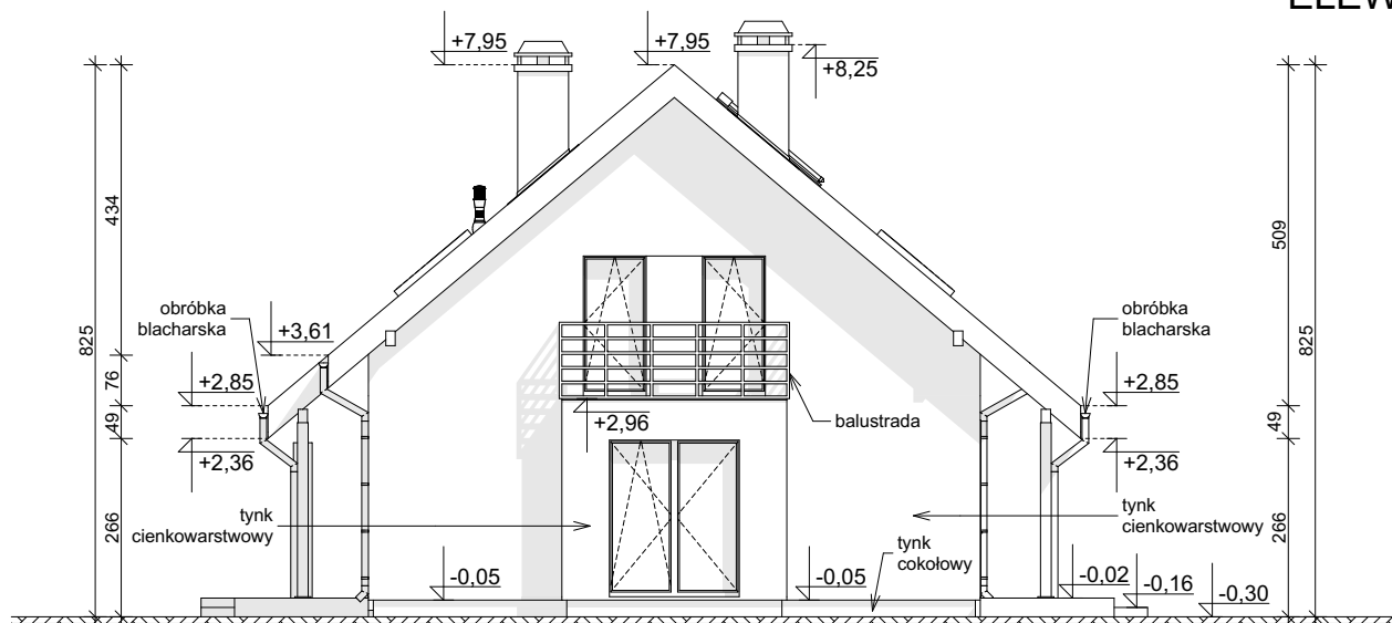
ELEVACJA BOCZNA
