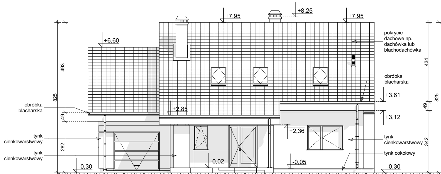
ELEWACJA FRONTOWA
