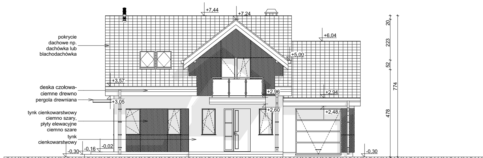
ELEWACJA FRONTOWA
