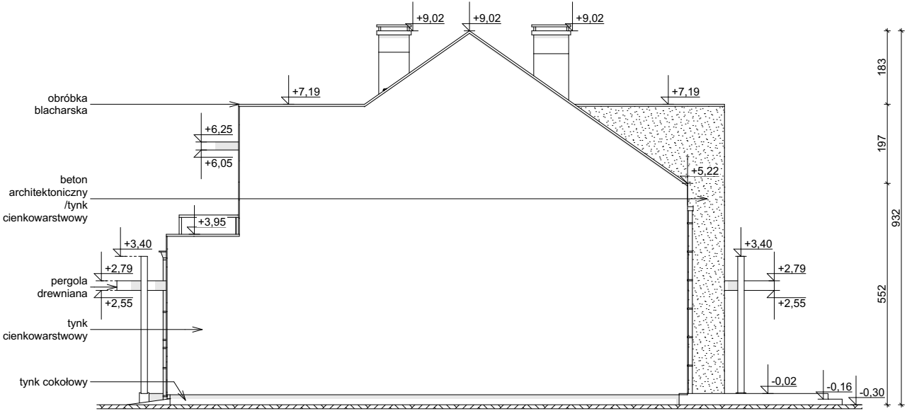
ELEWACJA BOCZNA
