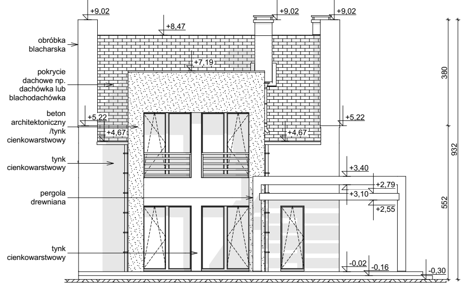
ELEWACJA OGRODOWA
