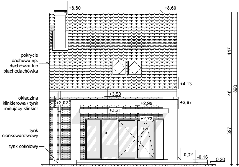
ELEWACJA OGRODOWA
