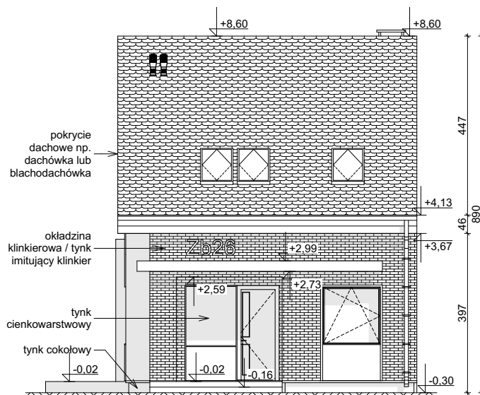
ELEWACJA FRONTOWA
