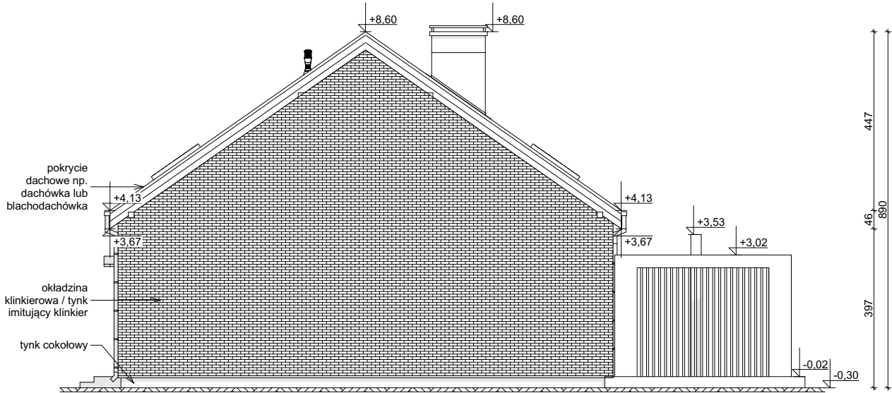
ELEWACJA BOCZNA
