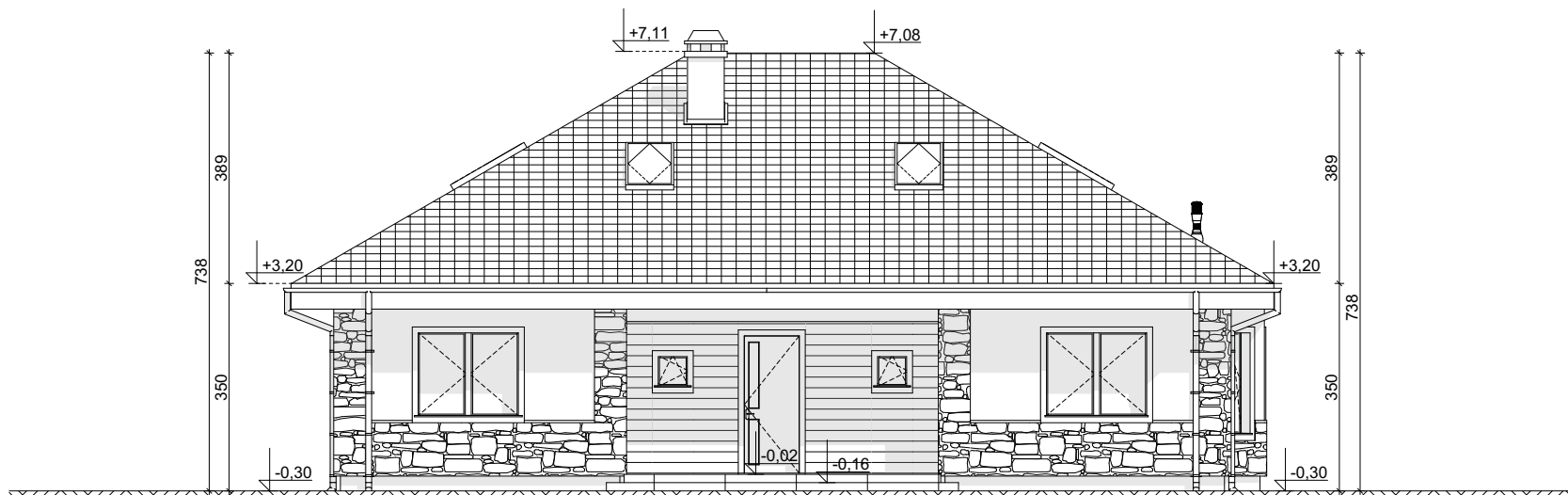
ELEWACJA FRONTOWA
