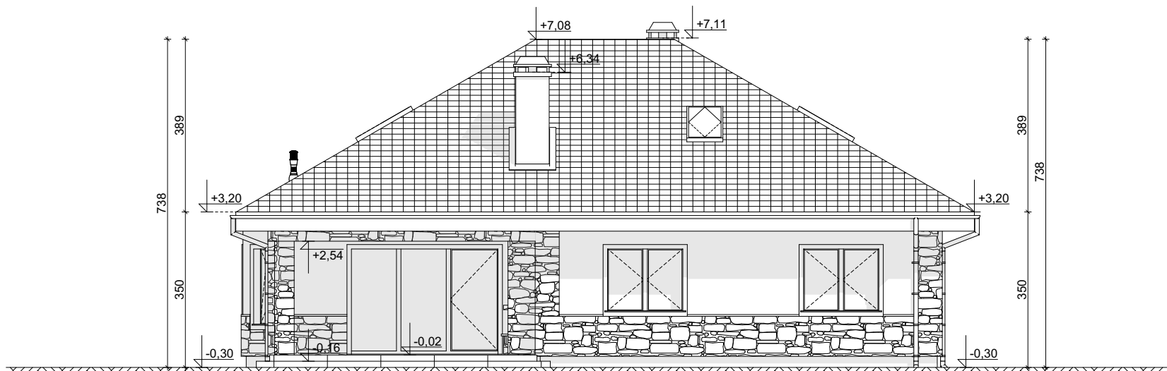
ELEWACJA BOCZNA
