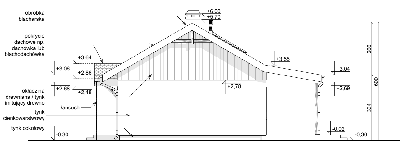
ELEWACJA BOCZNA
