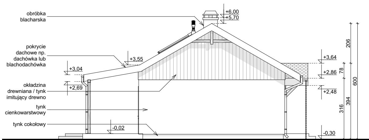
ELEWACJA BOCZNA
