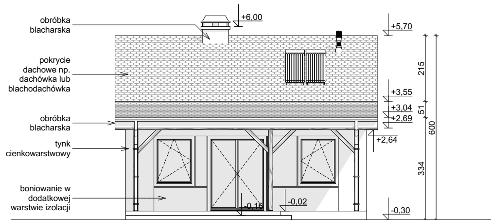
ELEWACJA OGRODOWA
