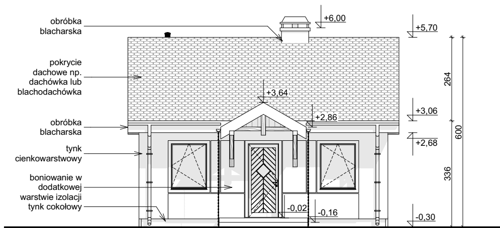
ELEWACJA FRONTOWA
