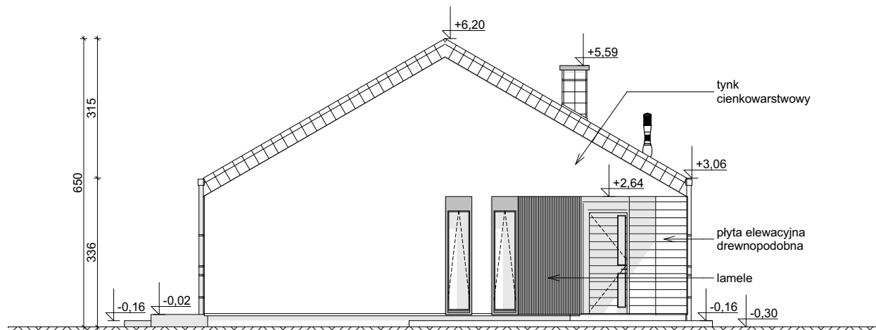
ELEWACJA FRONTOWA
