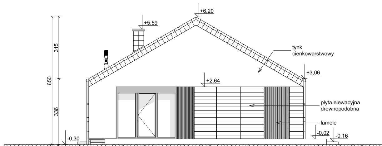
ELEWACJA OGRODOWA
