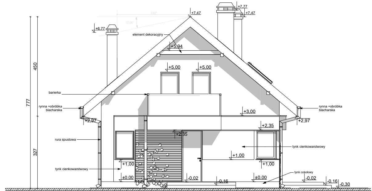
ELEWACJA FRONTOWA
