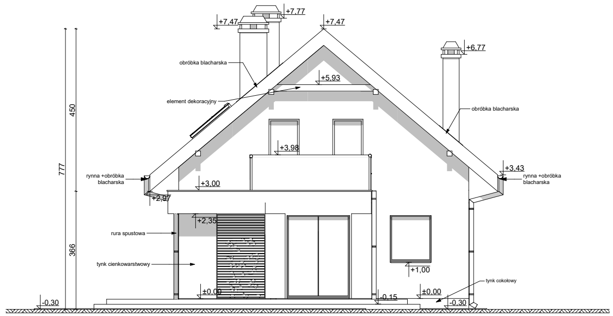
ELEWACJA TYLNA
