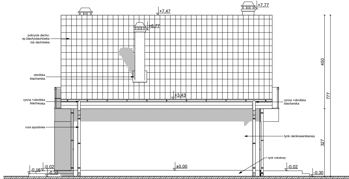
ELEWACJA BOCZNA
