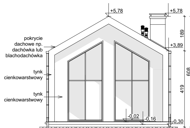
ELEWACJA OGRODOWA
