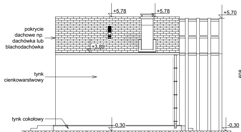
ELEWACJA BOCZNA
