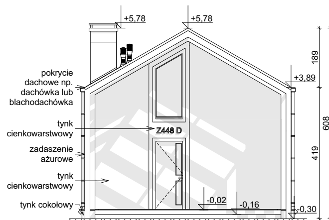
ELEWACJA FRONTOWA
