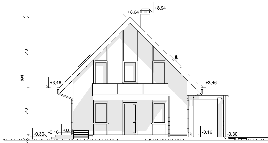
ELEWACJA FRONTOWA
