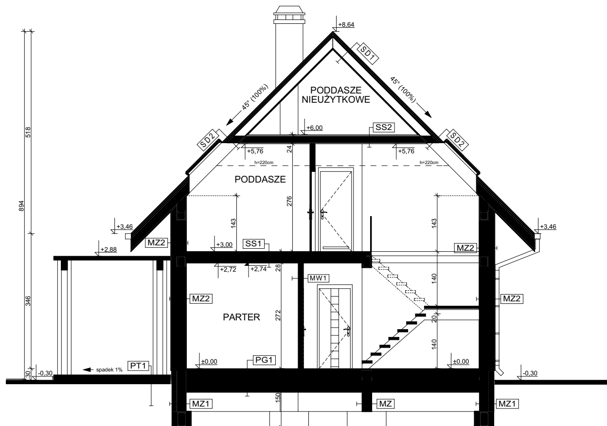
PRZEKRÓJ A-A
