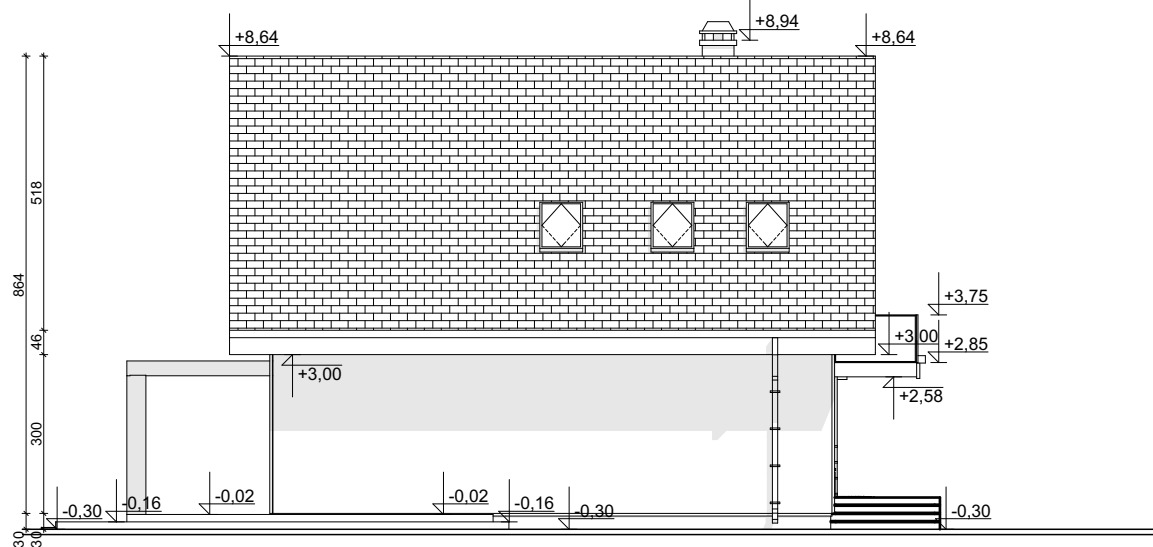
ELEWACJA BOCZNA
