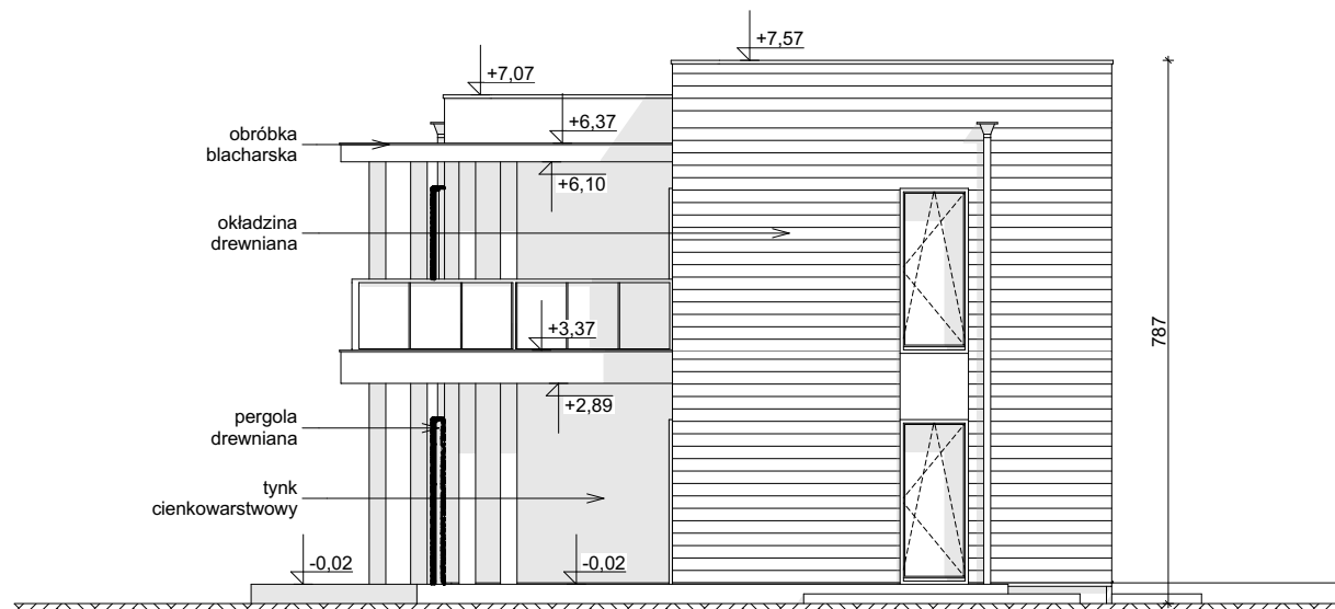
ELEWACJA BOCZNA
