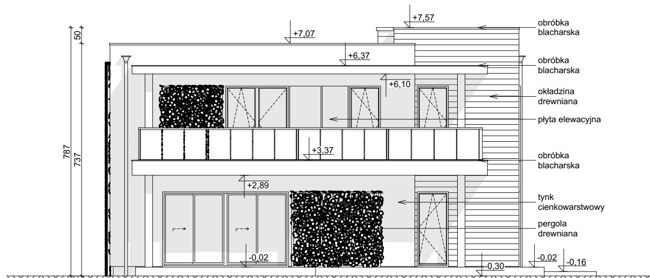
ELEWACJA OGRODOWA
