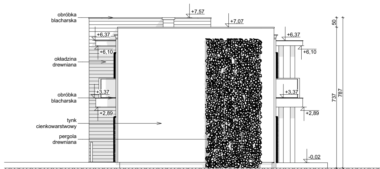
ELEWACJA BOCZNA
