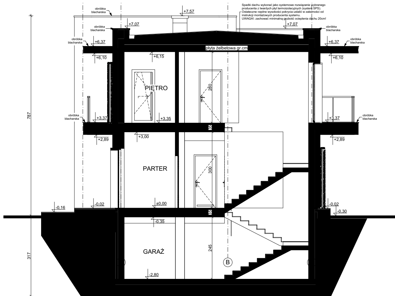
B-B PRZEKRÓJ
