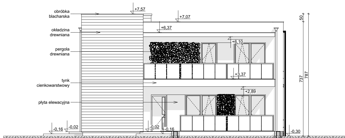
ELEWACJA FRONTOWA
