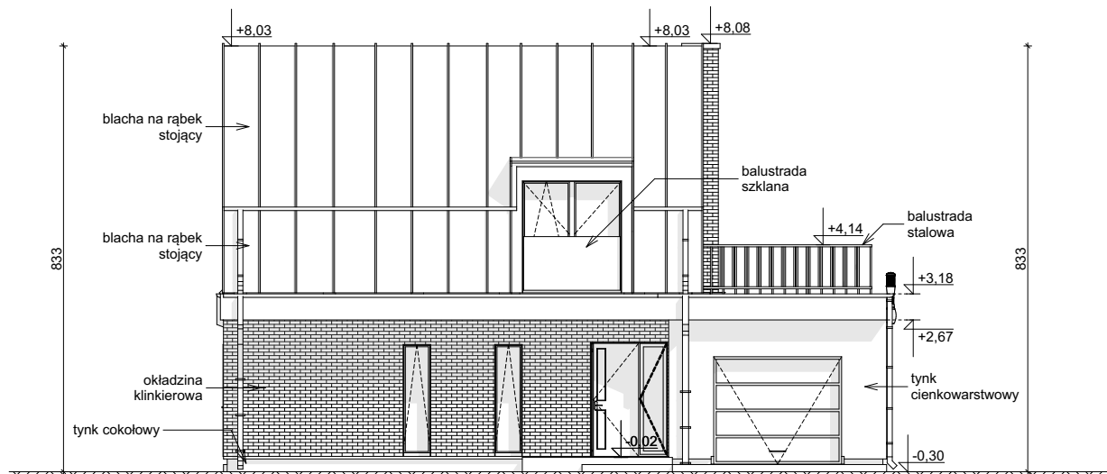
ELEWACJA FRONTOWA
