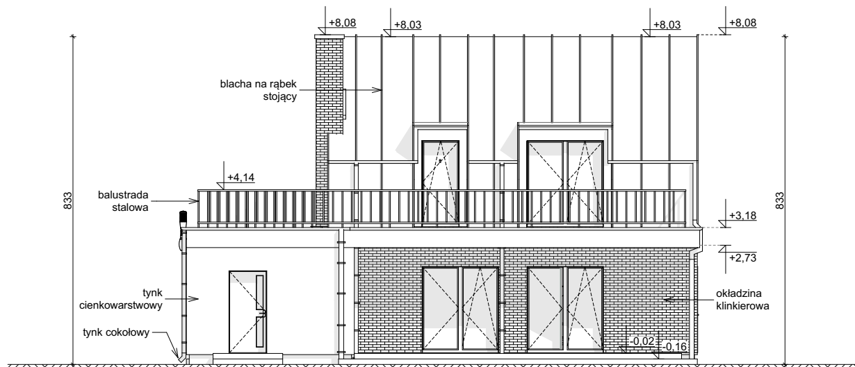
ELEWACJA OGRODOWA
