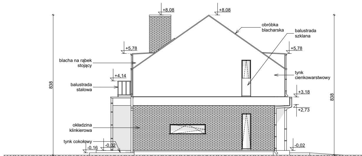
ELEWACJA BOCZNA
