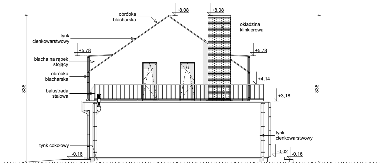
ELEWACJA BOCZNA
