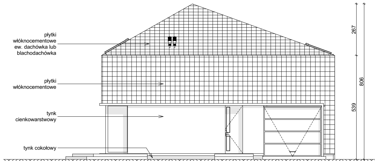
ELEWACJA FRONTOWA
