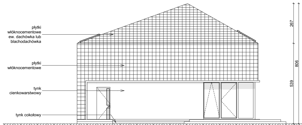
ELEWACJA OGRODOWA
