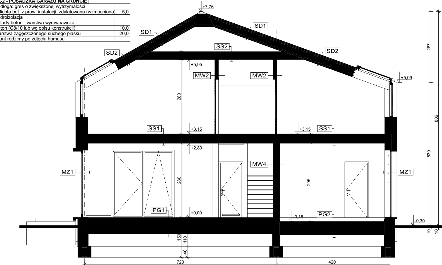
A-A Przekrój
