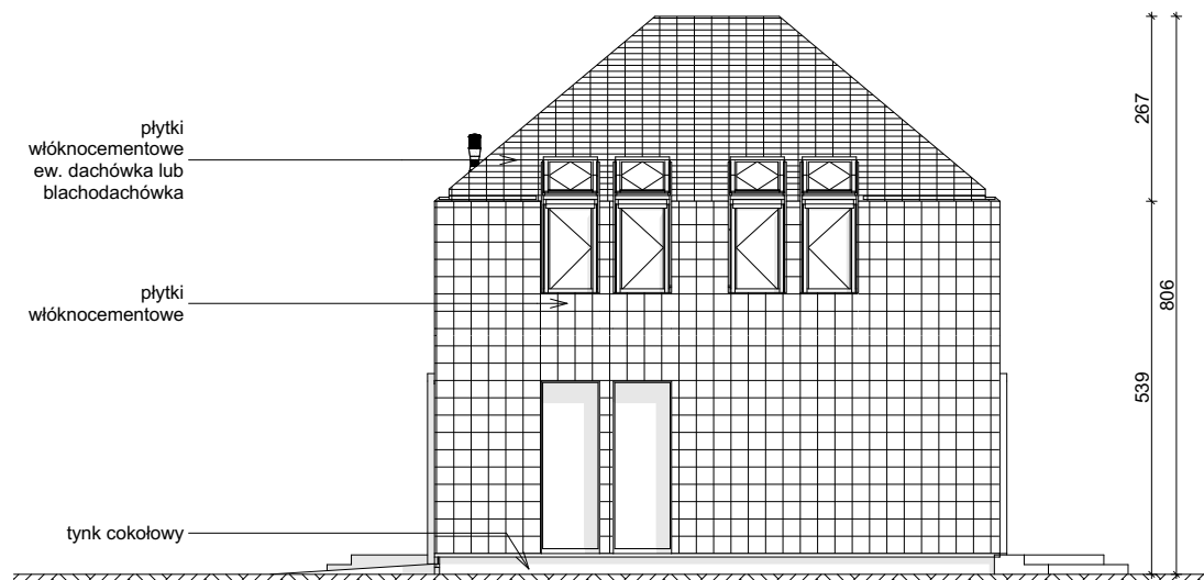
ELEWACJA BOCZNA
