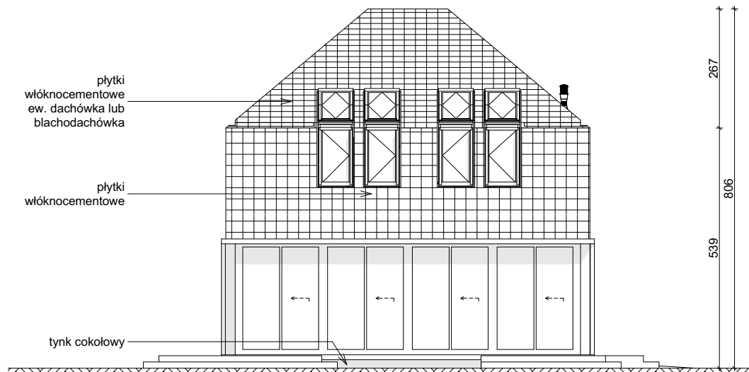
ELEWACJA BOCZNA
