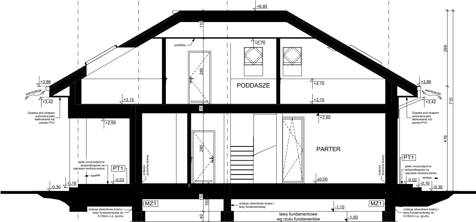
B-B PRZEKRÓJ
