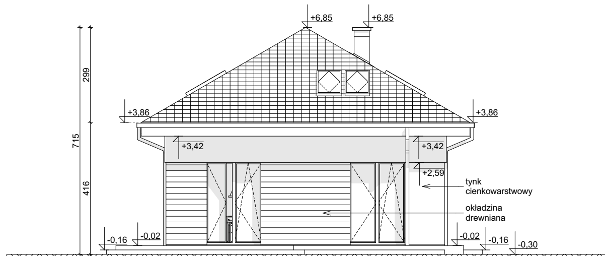
ELEWACJA OGRODOWA
