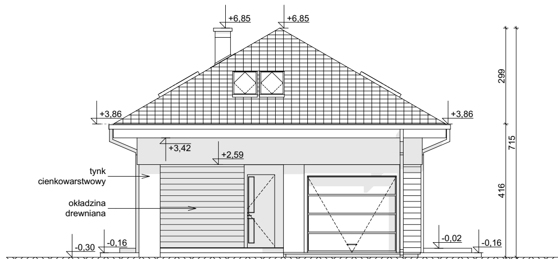
ELEWACJA FRONTOWA
