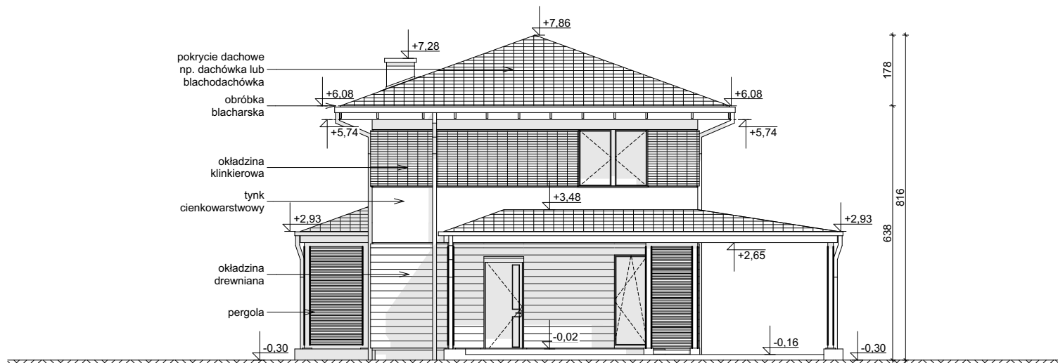
ELEWACJA FRONTOWA
