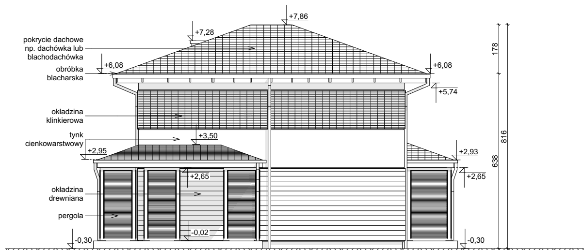
ELEWACJA BOCZNA
