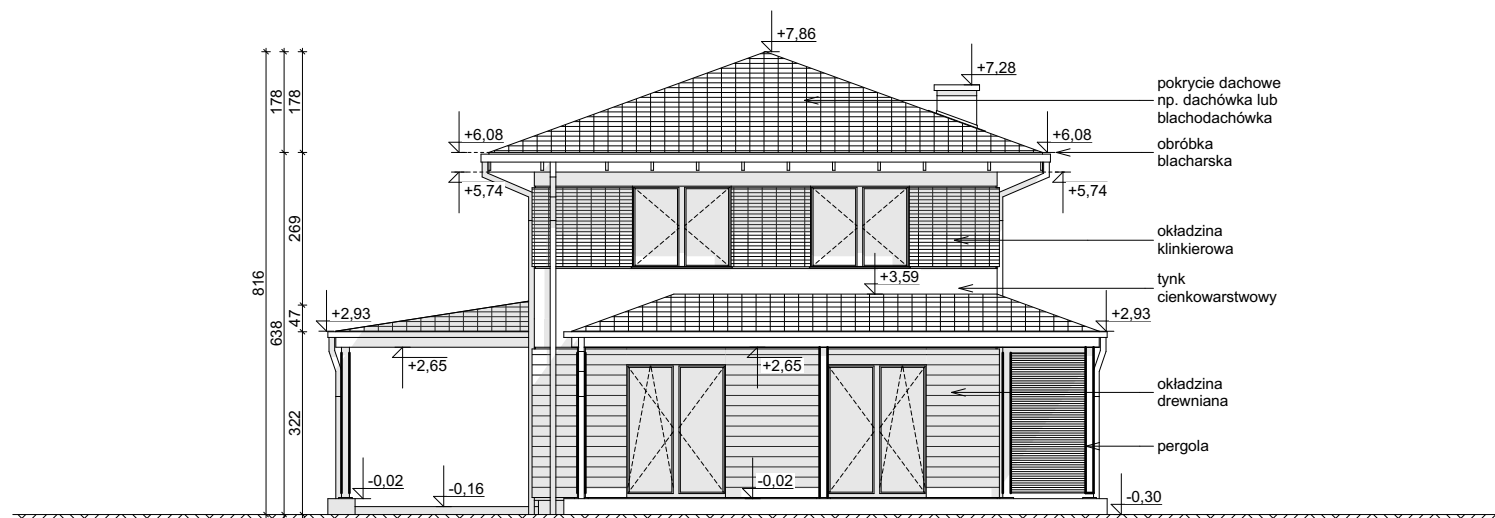
ELEWACJA OGRODOWA
