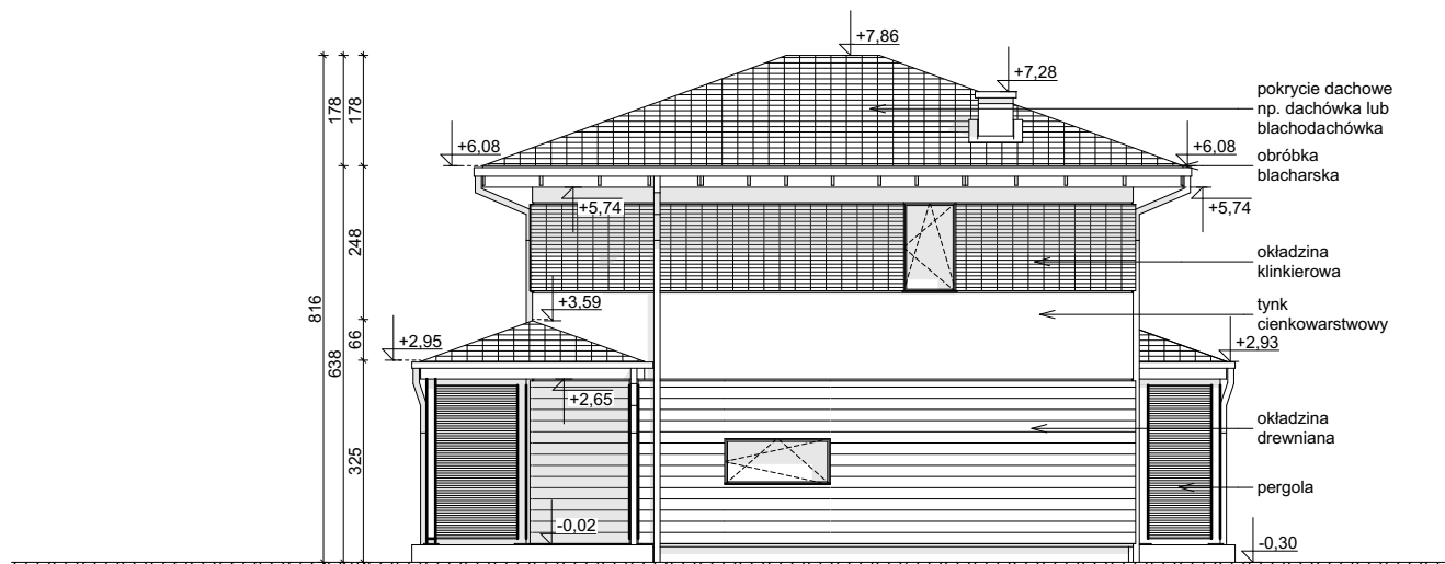
ELEWACJA BOCZNA
