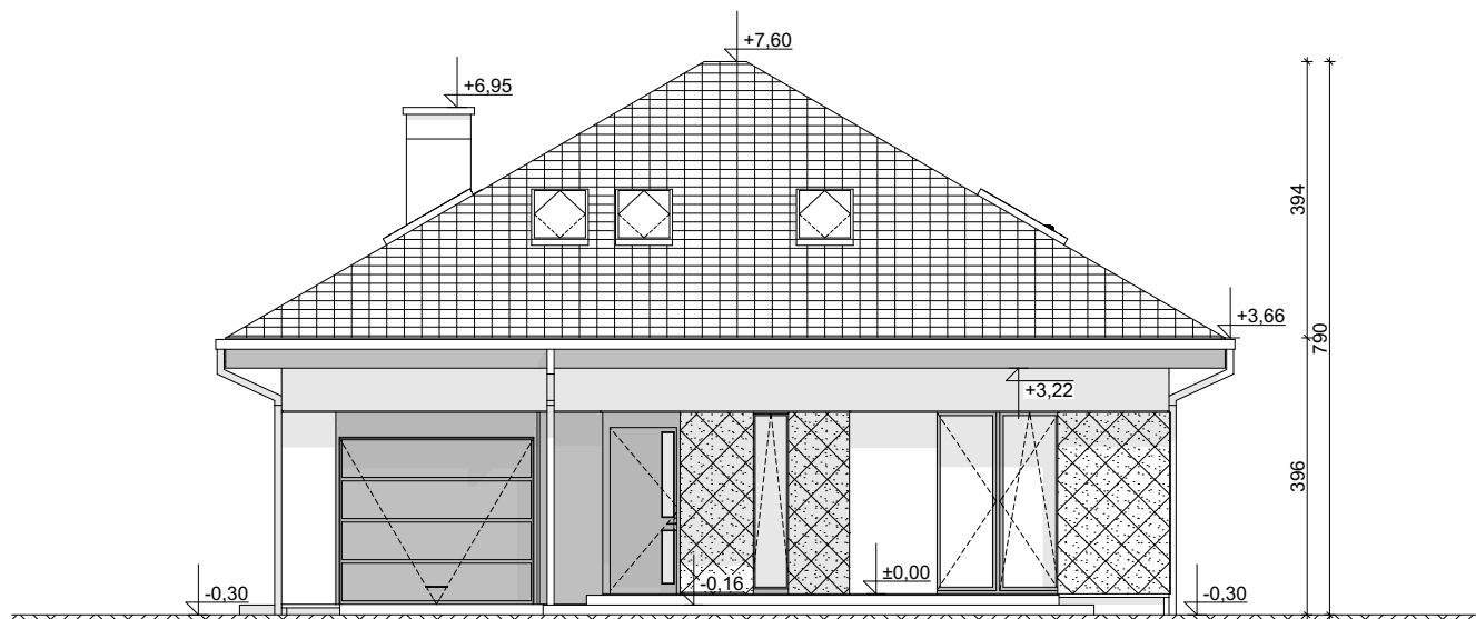
ELEWACJA FRONTOWA
