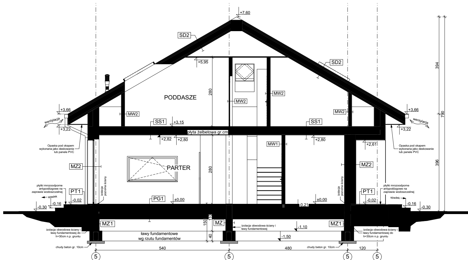
B-B PRZEKRÓJ
