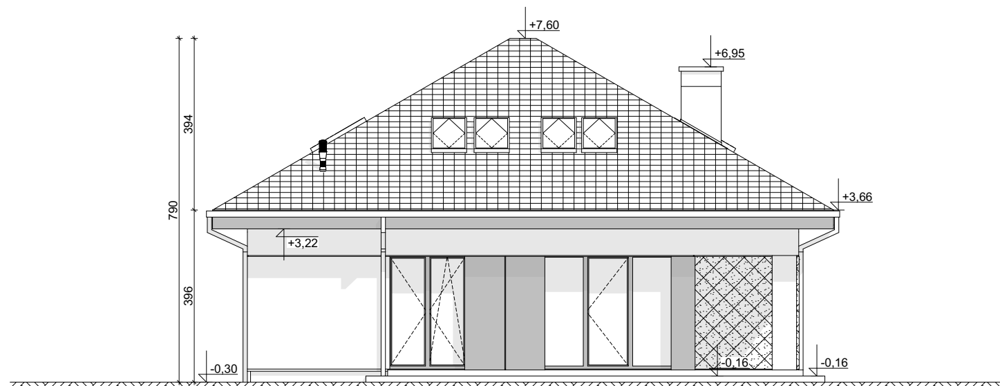
ELEWACJA OGRODOWA
