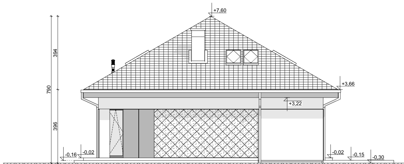
ELEWACJA BOCZNA
