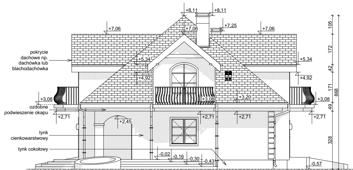
ELEWACJA BOCZNA
