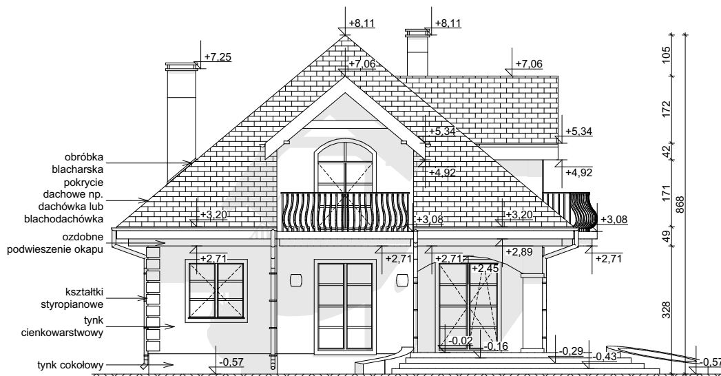
ELEWACJA OGRODOWA
