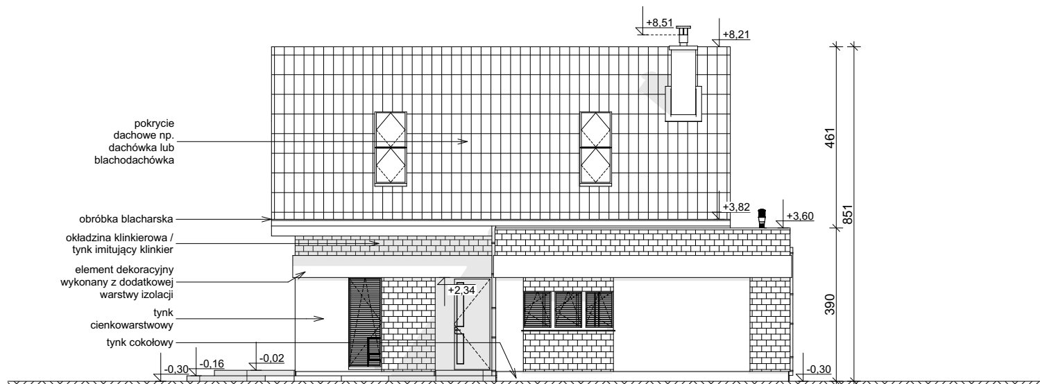
ELEWACJA FRONTOWA
