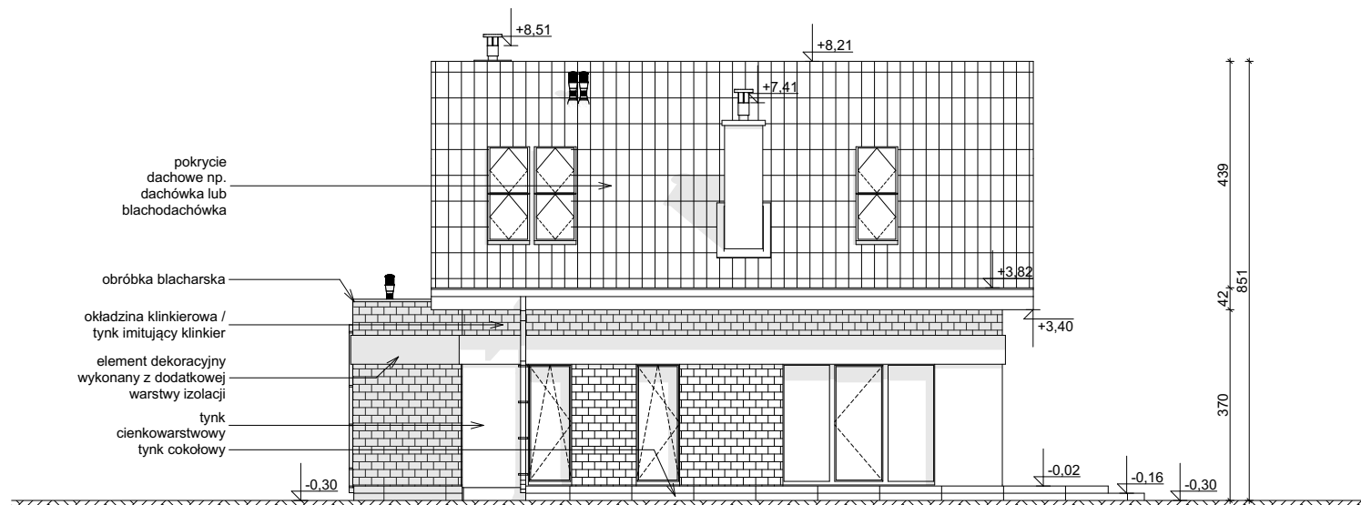
ELEWACJA OGRODOWA
