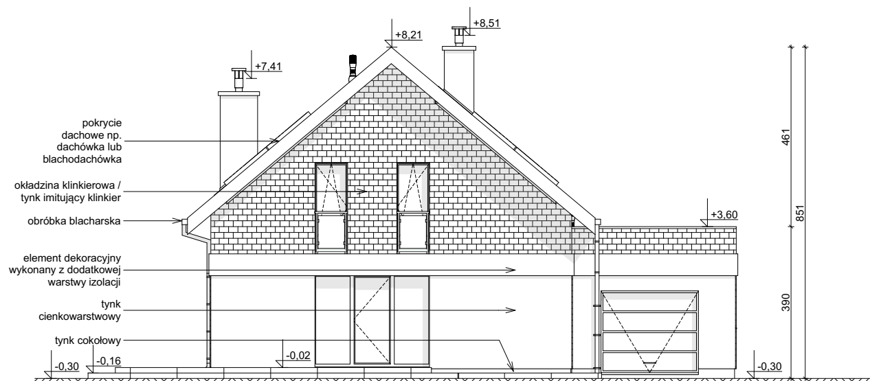
ELEWACJA BOCZNA
