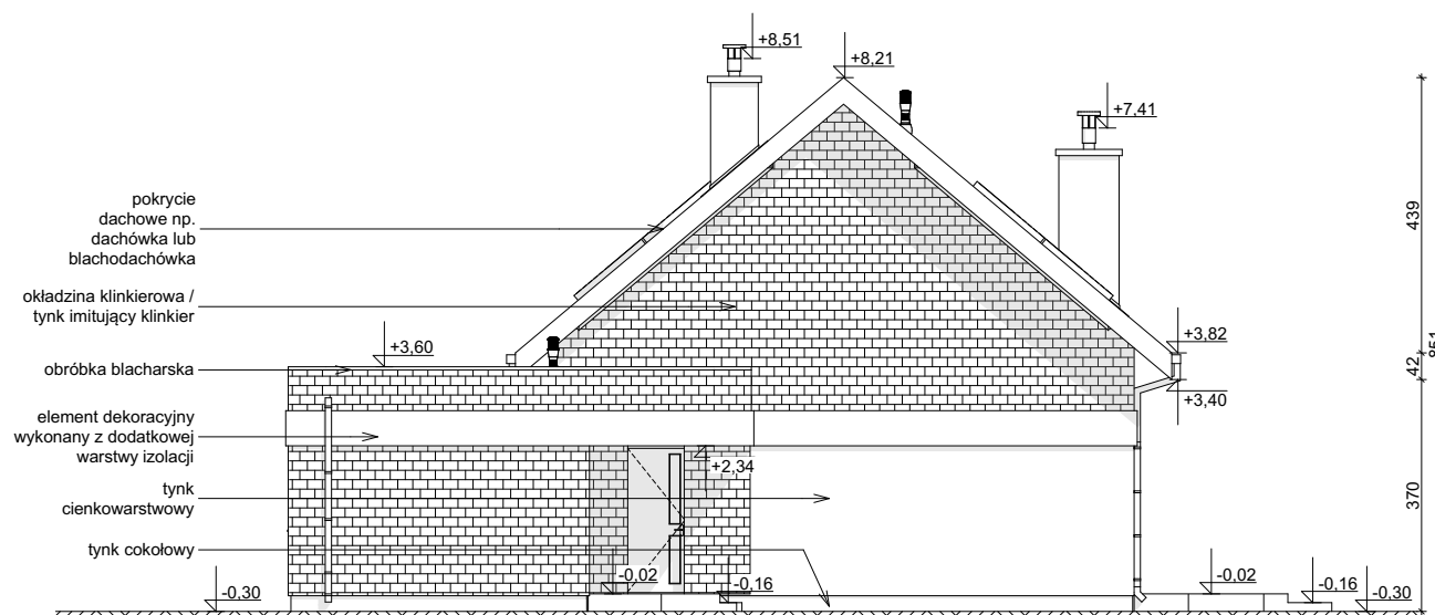
ELEWACJA BOCZNA
