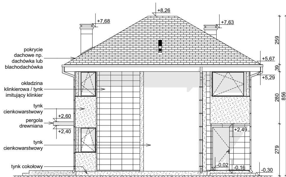
ELEWACJA BOCZNA
