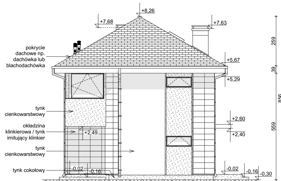
ELEWACJA FRONTOWA
