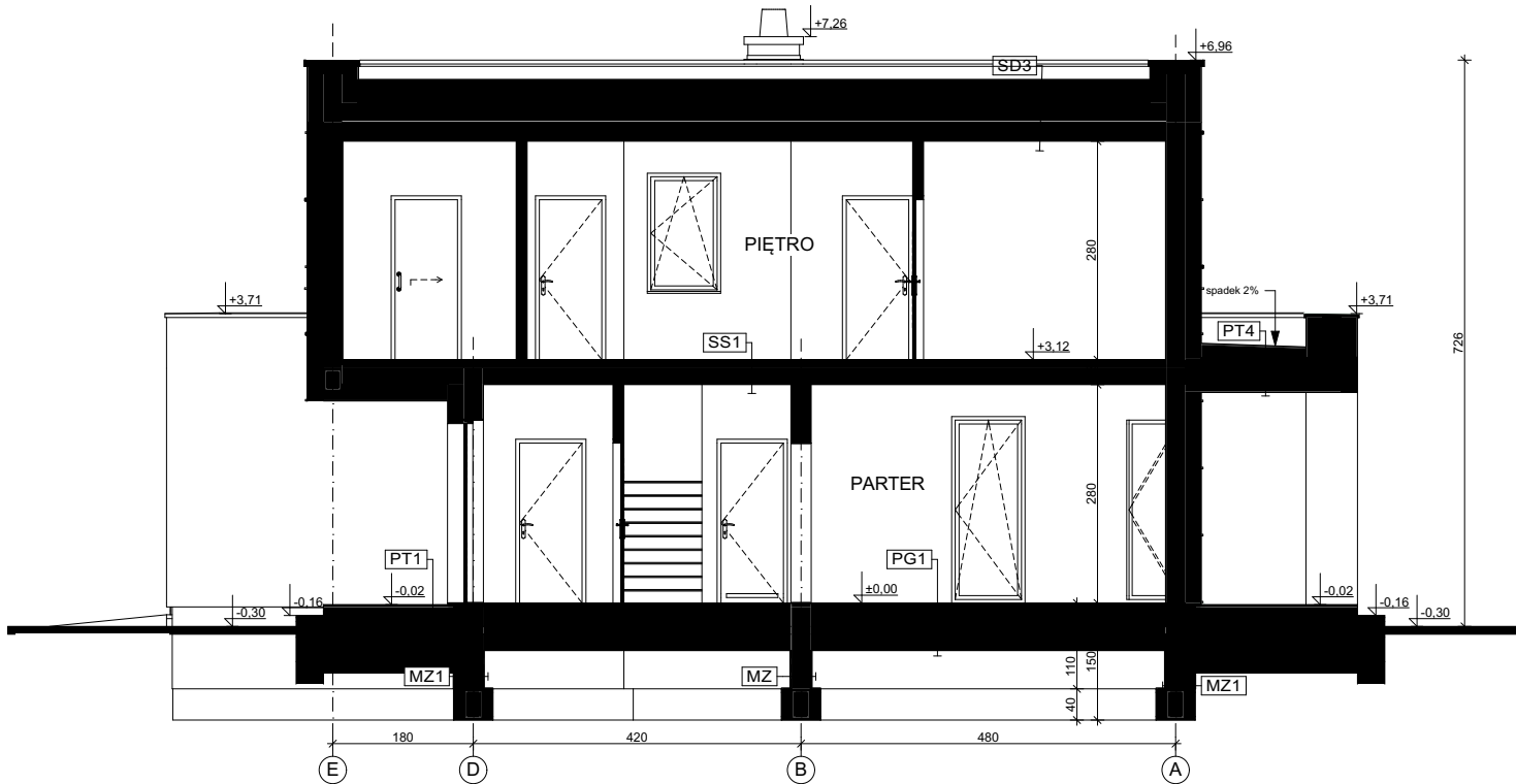
B-B PRZEKRÓJ
