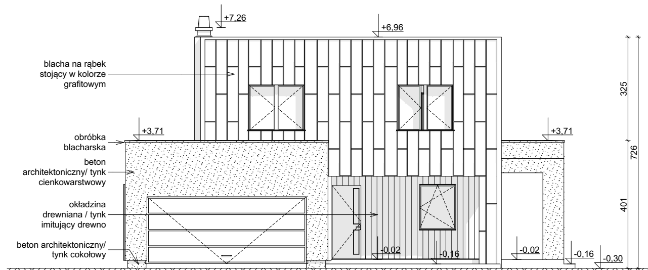
ELEWACJA FRONTOWA
