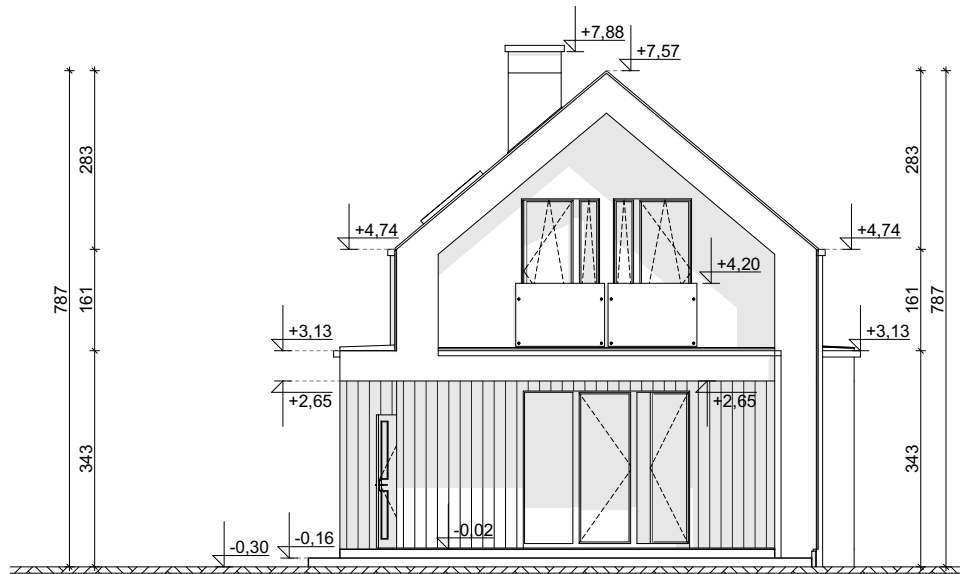
ELEWACJA OGRODOWA
