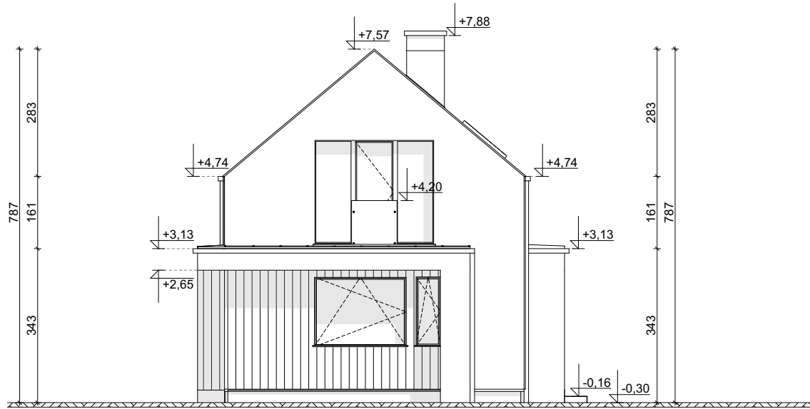
ELEWACJA FRONTOWA
