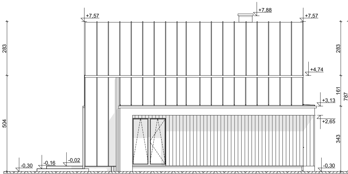
ELEWACJA BOCZNA
