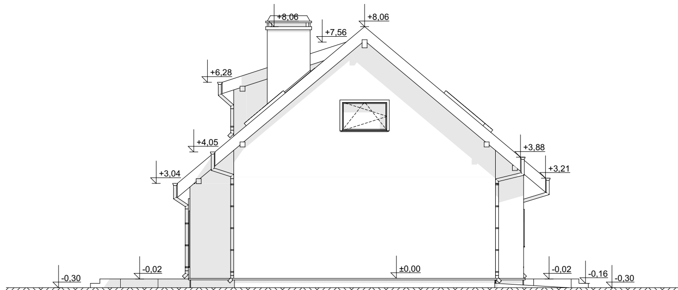
ELEVACJA BOCZNA
