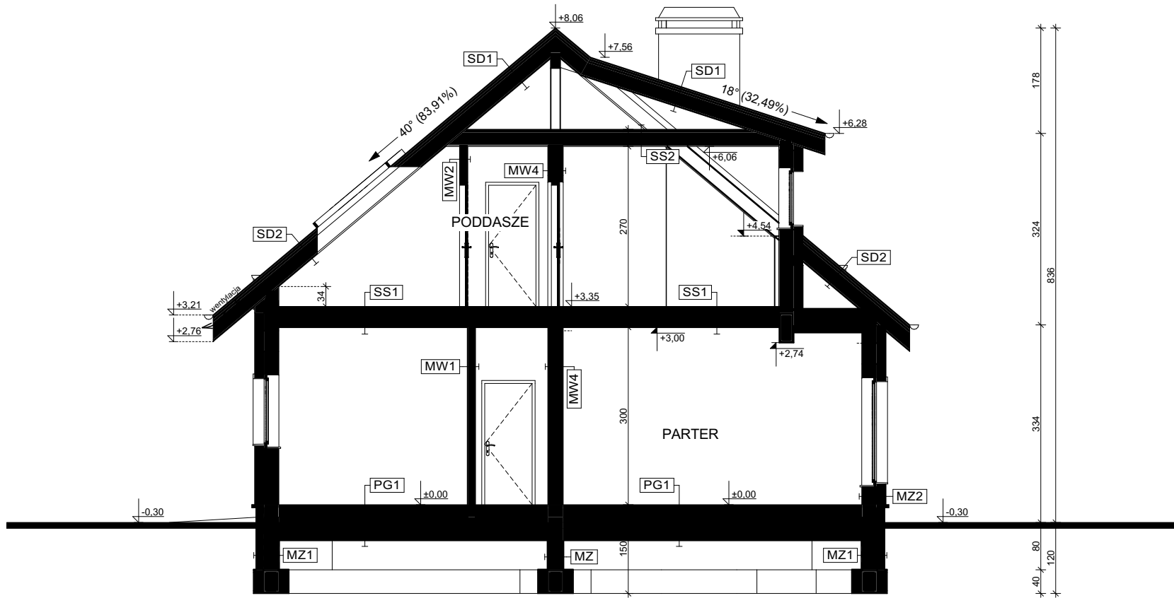
PRZEKRÓJ B-B
