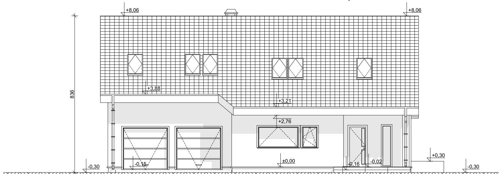
ELEVACJA FRONTOWA
