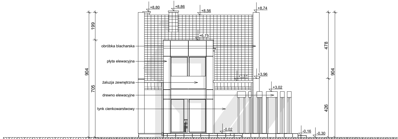
ELEWACJA OGRODOWA
