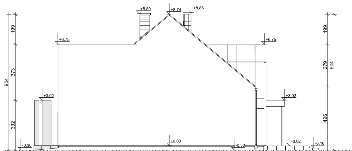
ELEWACJA BOCZNA
