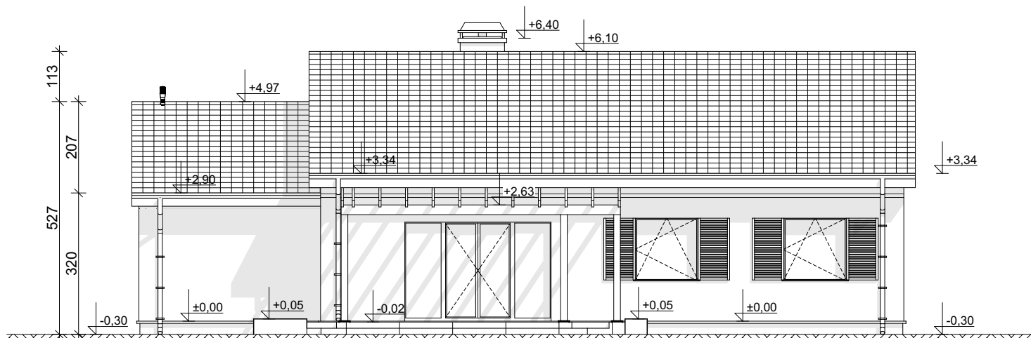
ELEWACJA OGRODOWA
