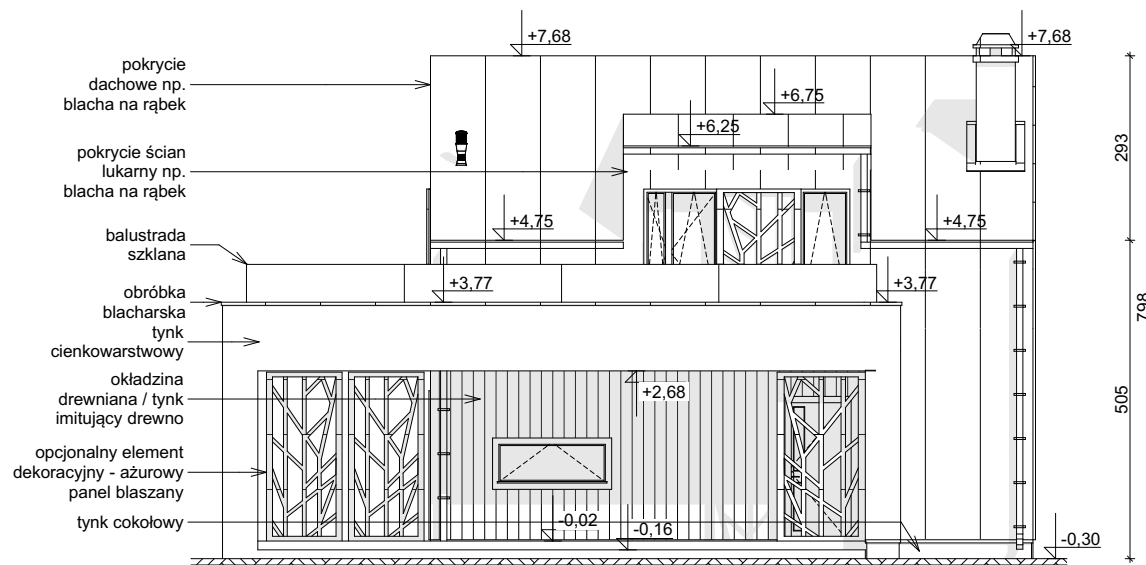
ELEWACJA FRONTOWA
