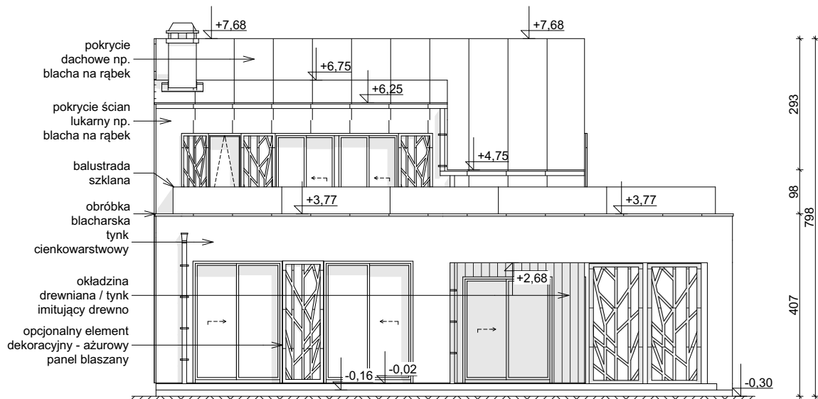
ELEWACJA OGRODOWA
