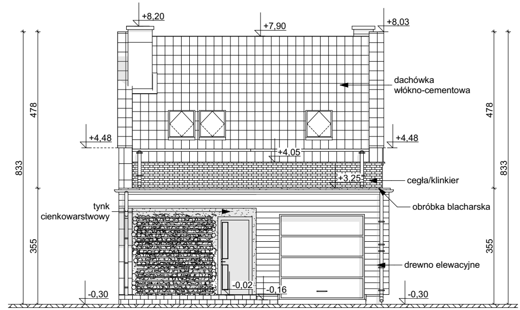
ELEWACJA FRONTOWA
