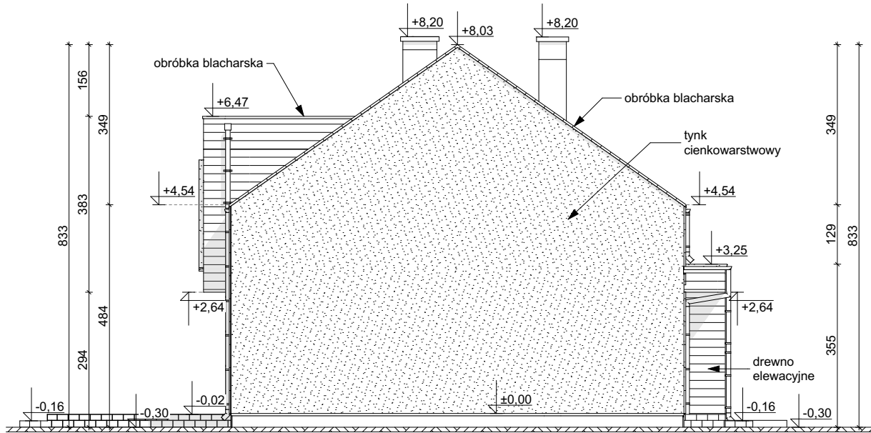
ELEWACJA BOCZNA
