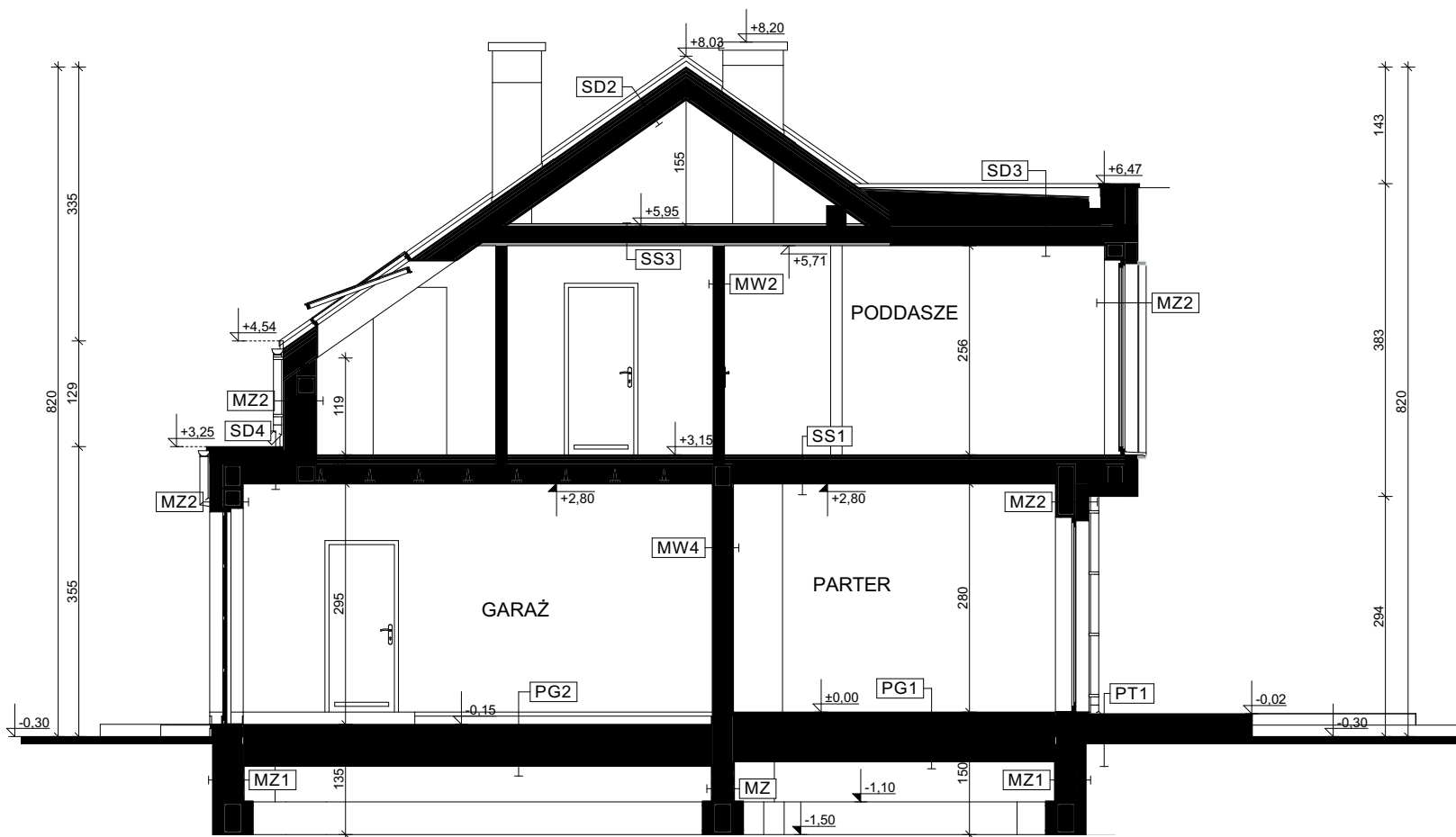
B-B PRZEKRÓJ
