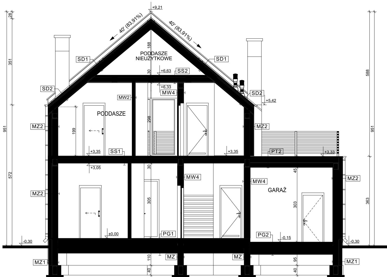
PRZEKRÓJ A-A
