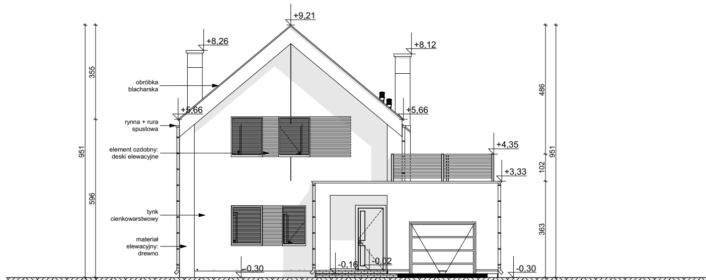
ELEWACJA FRONTOWA
