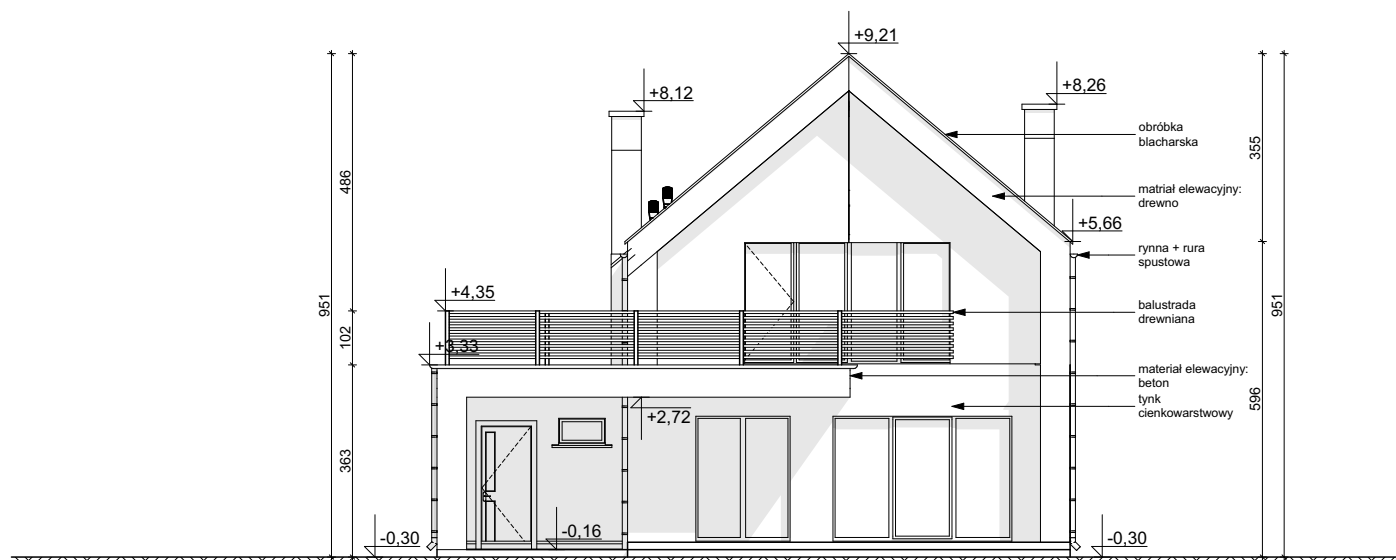
ELEWACJA OGRODOWA
