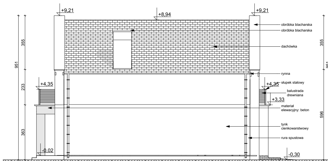
ELEWACJA BOCZNA
