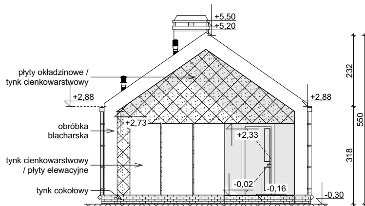
ELEWACJA FRONTOWA
