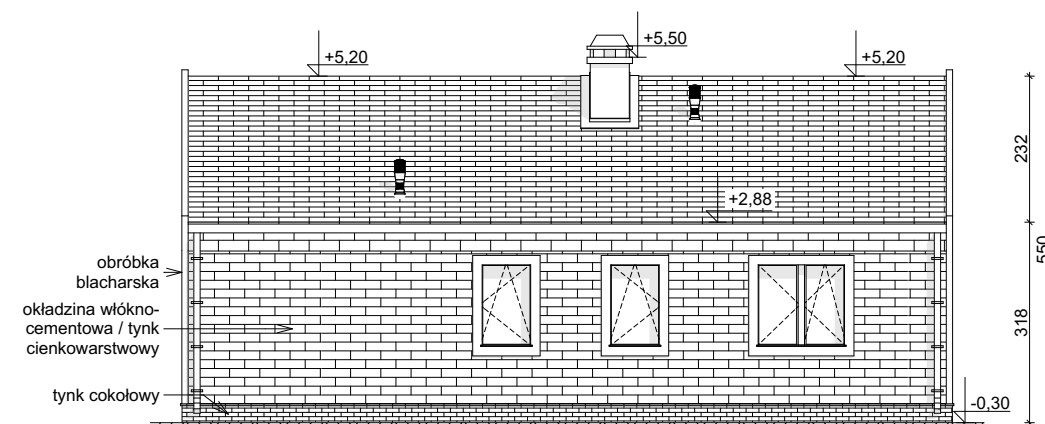
ELEWACJA BOCZNA
