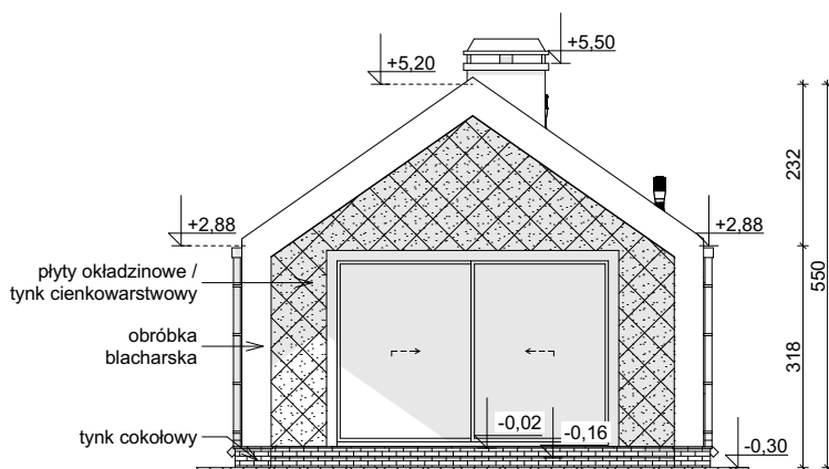
ELEWACJA OGRODOWA
